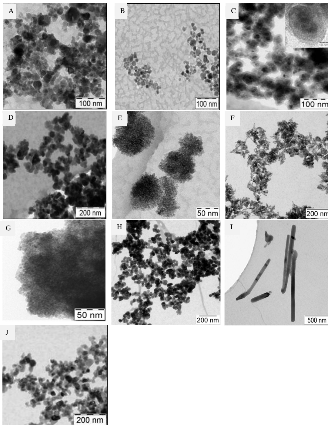
Figure S2. TEM analysis of ZnO nanoparticles. TEM micrographs of A) ZnO-1, B) ZnO-2, C) ZnO-3, D) ZnO-4, E) ZnO-5, F) ZnO-6, G) ZnO-7, H) ZnO-8, I) ZnO-9 and J) TiO 2 .
