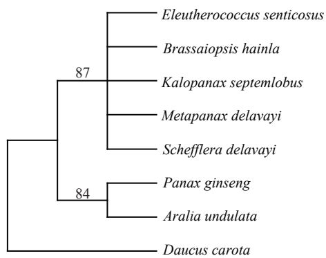
ycf3-trnS(GGA)
