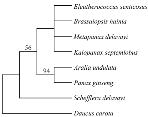
trnS(GCU)-trnG(UCC)
