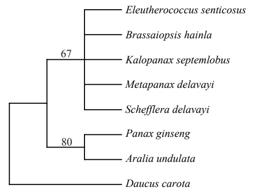
trnT(UGU)-trnL(UAA)
