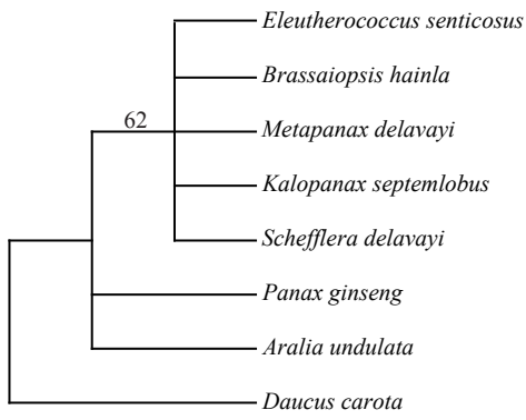
trnK(UUU)-rps16
