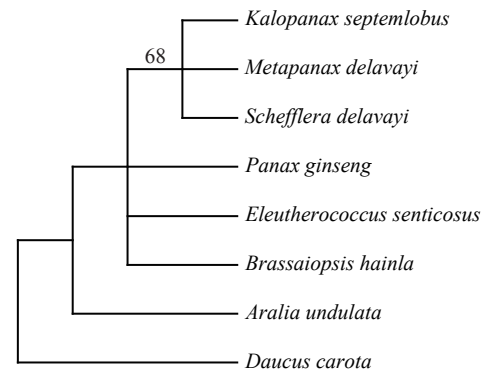
psbK-psbI
