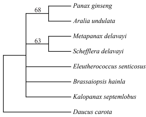
trnC(GCA)-petN
