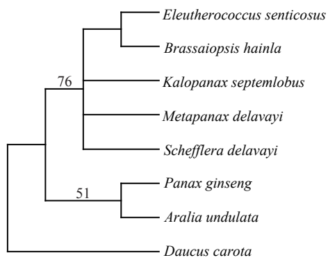
rpl32-trnL(UAG)
