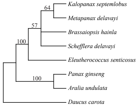
ycf1
