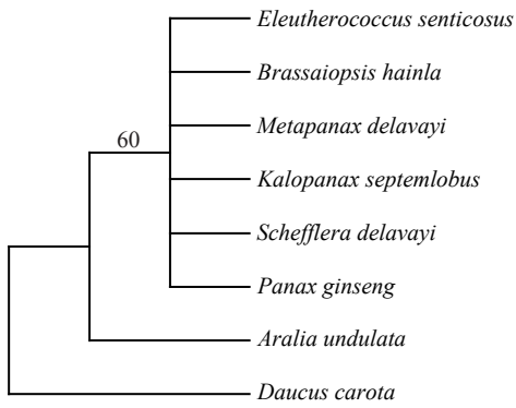
psaJ-rpl33
