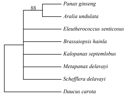
rps16-trnQ(UUG)
