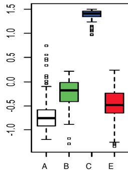
cluster VI (135)
