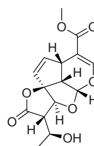
(IV) Allamandicin
