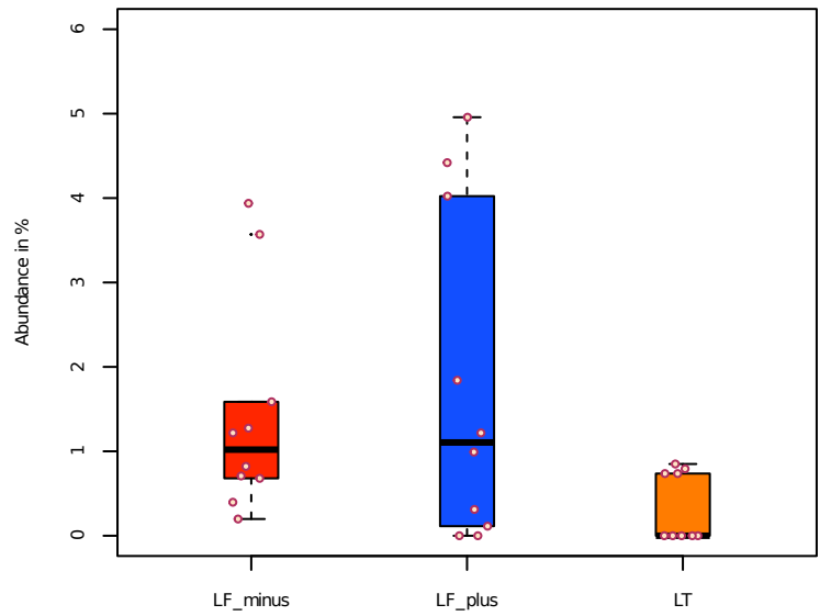
Pelomonas
