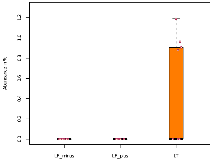
Brochothrix
