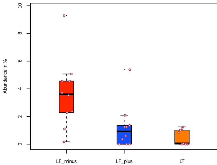
Polaromonas
