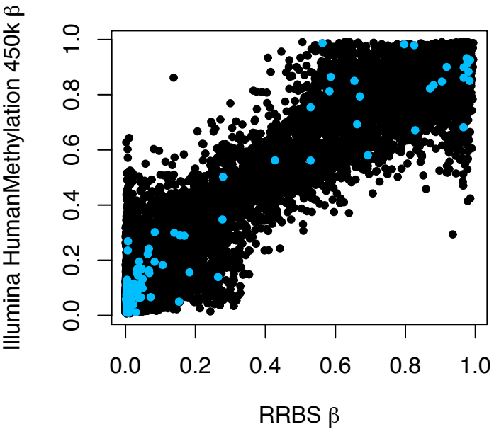
Dataset 1
