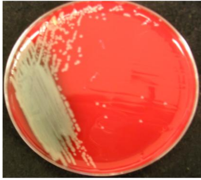
PAO1
