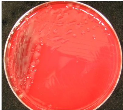
PA42
