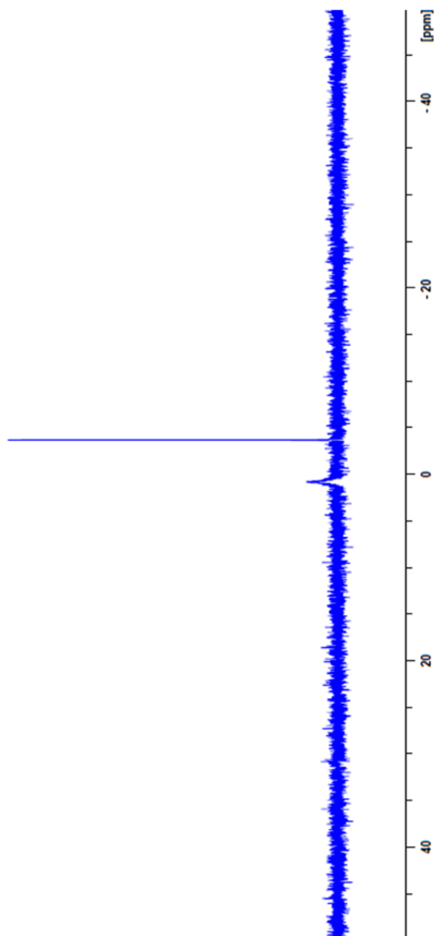
DSPE-PEG 2000 - TP
