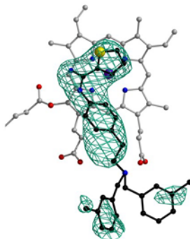
iNOS (mol.1)
