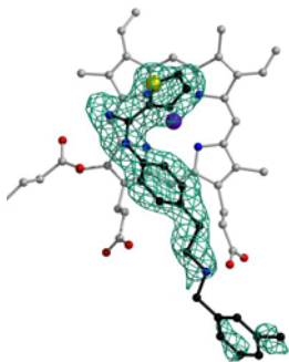
nNOS
