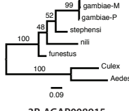
3R-AGAP008915
