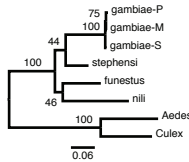
2R-AGAP002252
