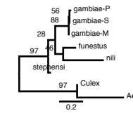
2R-AGAP001760
