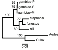
2R-AGAP002935
