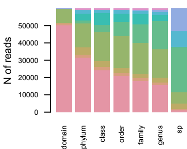
iMESS 1
