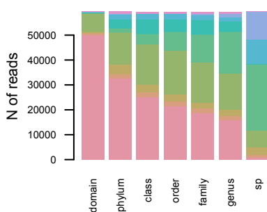
iMESS 2
