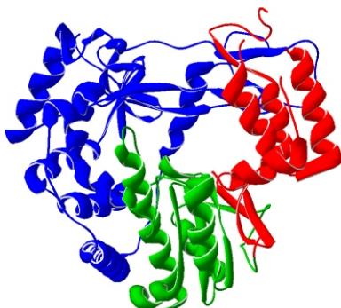
MuNORV1
