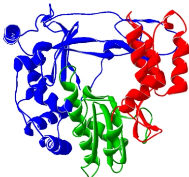
PoIV1
