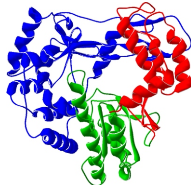
RHDV
