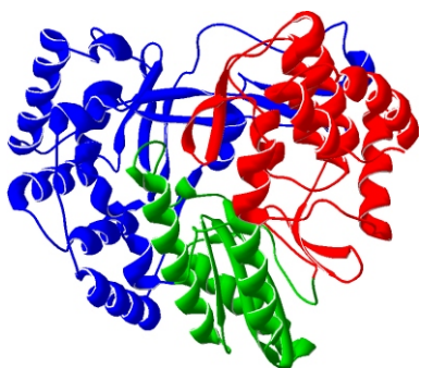
BVDV
