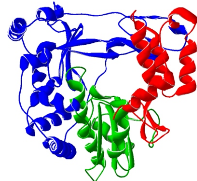
HuRV16
