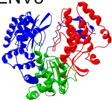
DENV3
