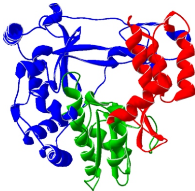
MuNORV1
