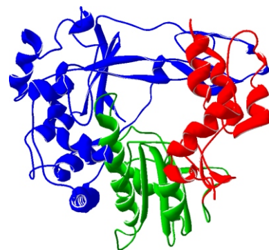
RHDV
