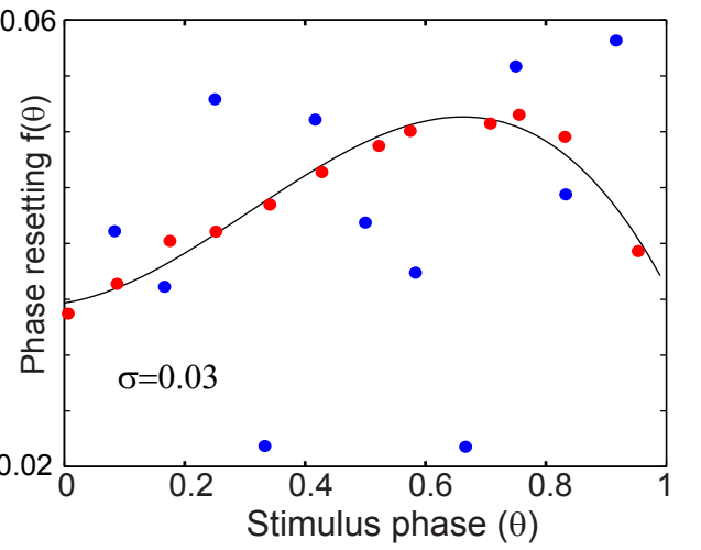
D2. PRC (high noise)
