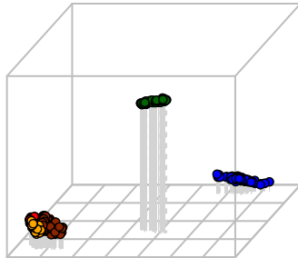
GC-MS
