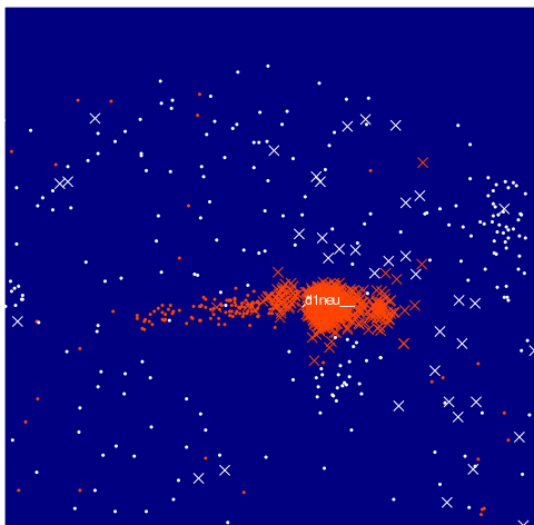
PSI-BLAST
