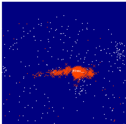
RankProp
