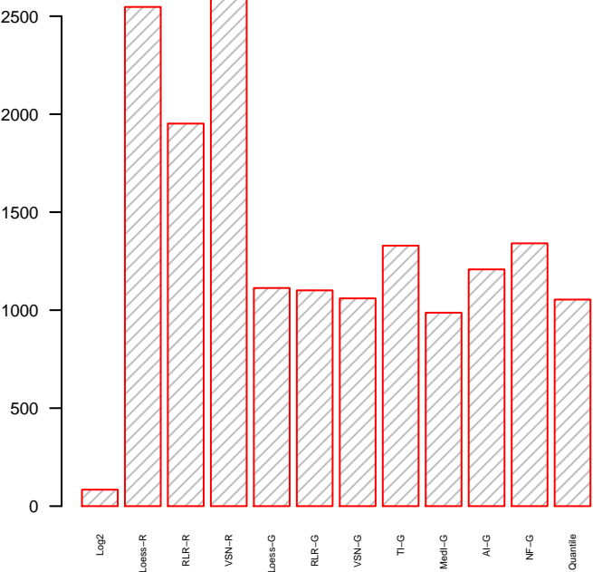
Kruskal Wallis
