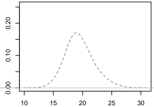
Quantile
