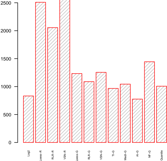
ANOVA
