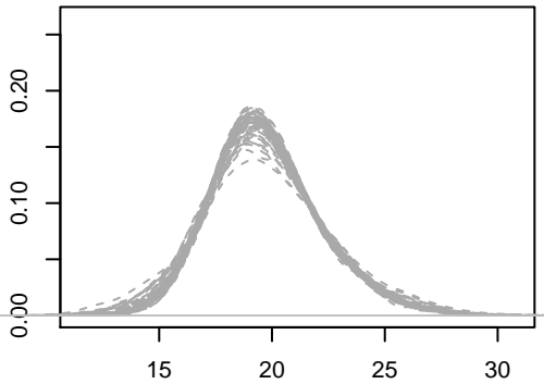
MedI-G
