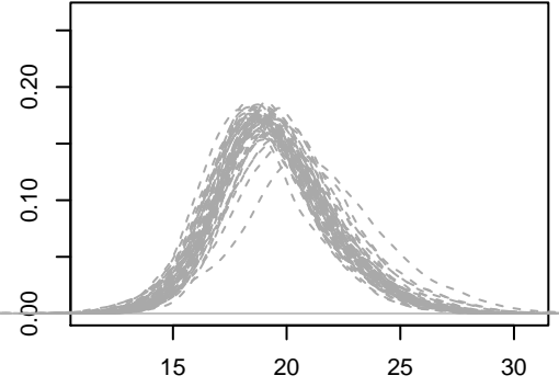
VSN-R
