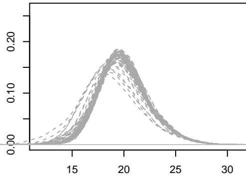
AI-G
