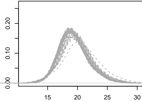
VSN-G
