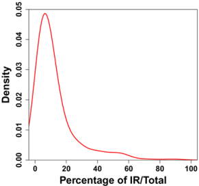
NaCl
