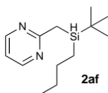
2-(( tert -Butyl(butyl)silyl)methyl)pyrimidine
