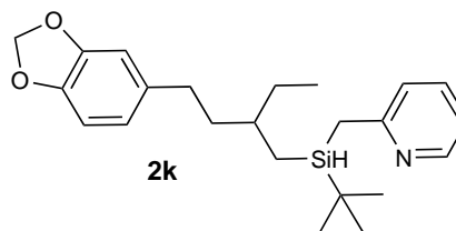
2-(((4-(Benzo[d][1,3]dioxol-5-yl)-2-ethylbutyl)( tert -butyl)silyl)methyl)pyridine
