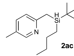
2-(( tert -Butyl(butyl)silyl)methyl)-4-methylpyridine
