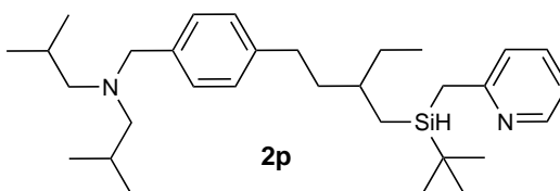
N -(4-(3-(( tert -Butyl(pyridin-2-ylmethyl)silyl)methyl)pentyl)benzyl)- N -isobutyl-2-methylpropan-1-amine
