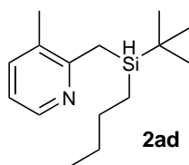
2-(( tert -Butyl(butyl)silyl)methyl)-3-methylpyridine
