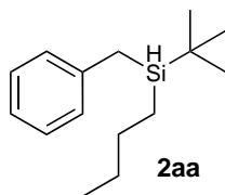
Benzyl( tert -butyl)(butyl)silane
