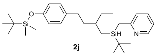
2-(( tert -Butyl(4-(4-( tert -butyl)dimethylsilyloxy)phenyl)-2-ethylbutyl)silyl)methyl)pyridine
