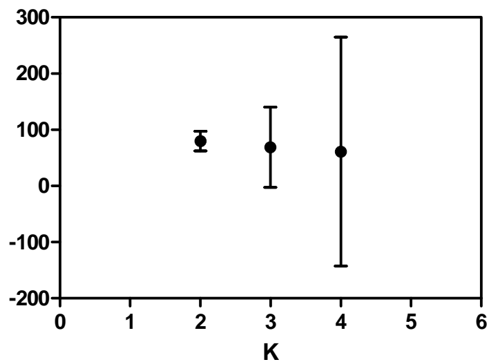
C. |\ln'' \Pr(X|K)|
