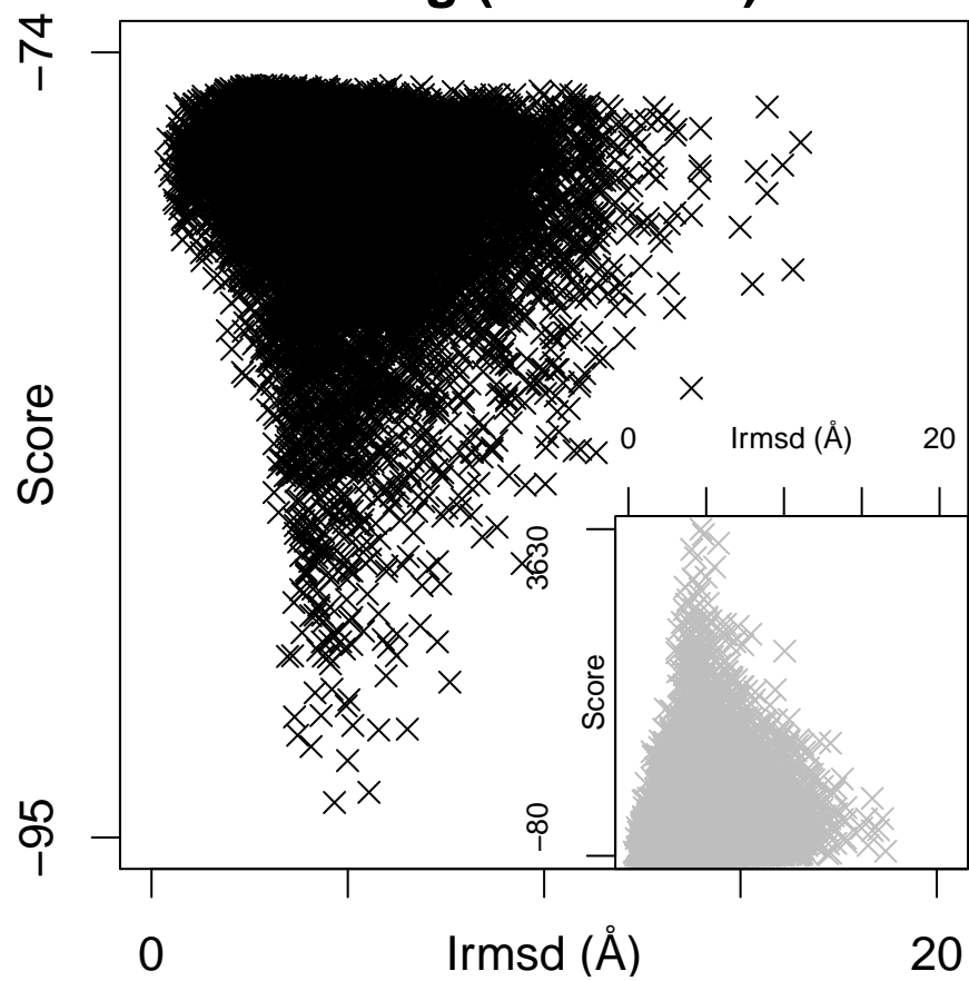
2err (ES = 2.48)
