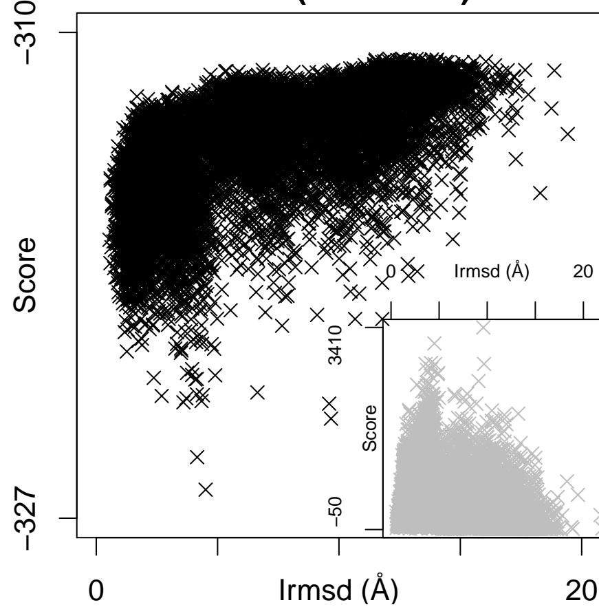
2ez6 (ES = 2.92)
