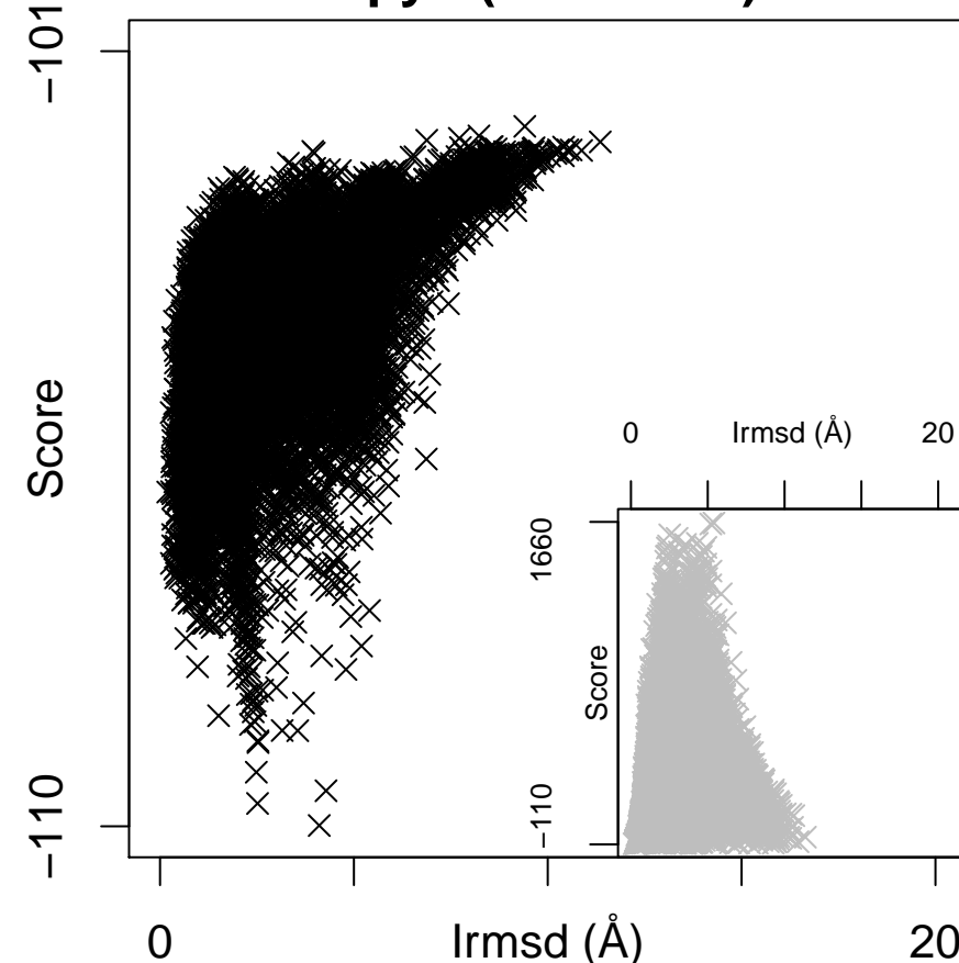
2py9 (ES = 2.95)
