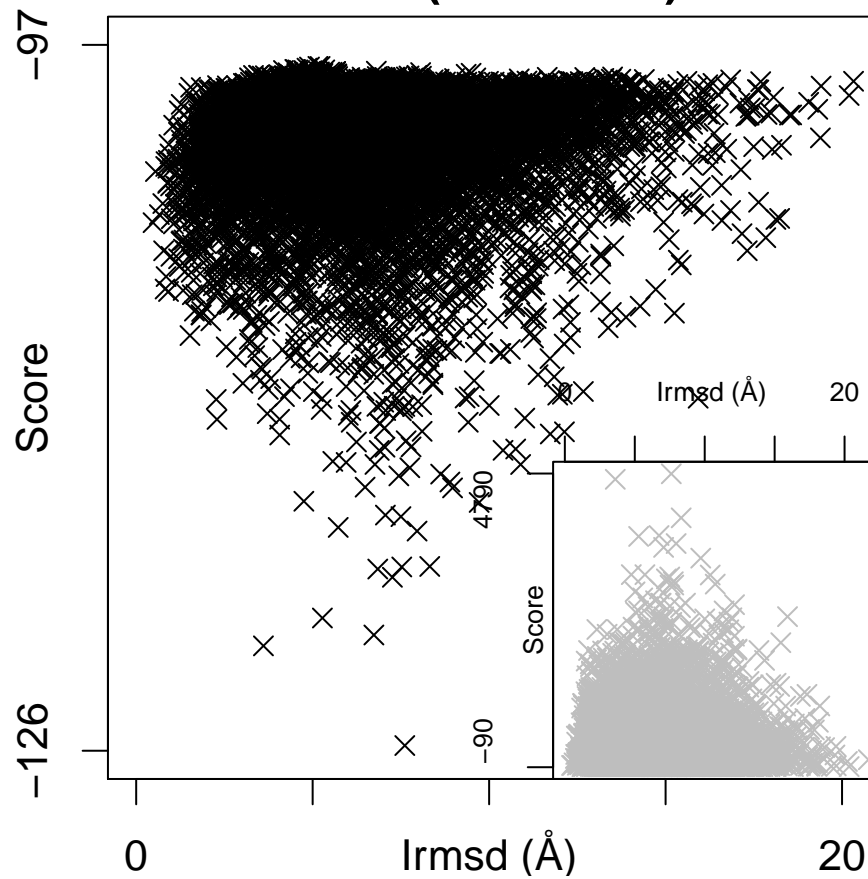
1ekz (ES = 0.81)
