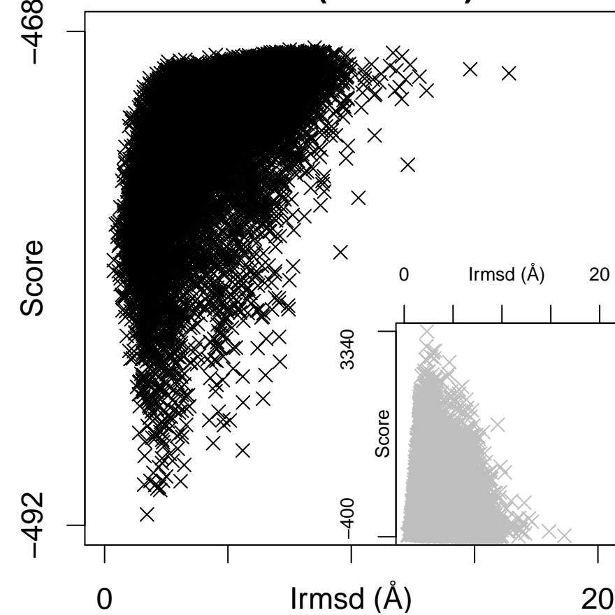
1hc8 (ES = 3.63)
