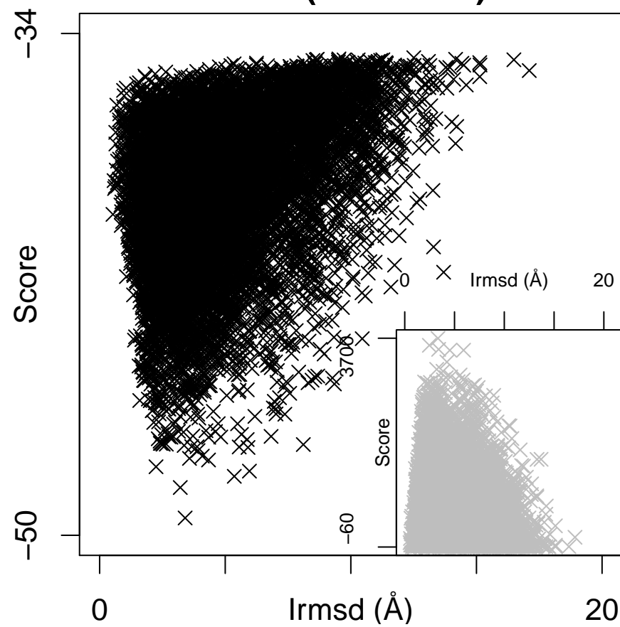
1ec6 (ES = 0.88)
