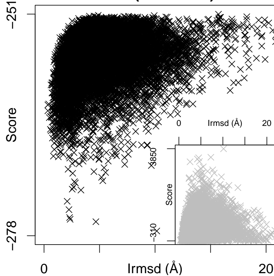
2ix1 (ES = 2.14)
