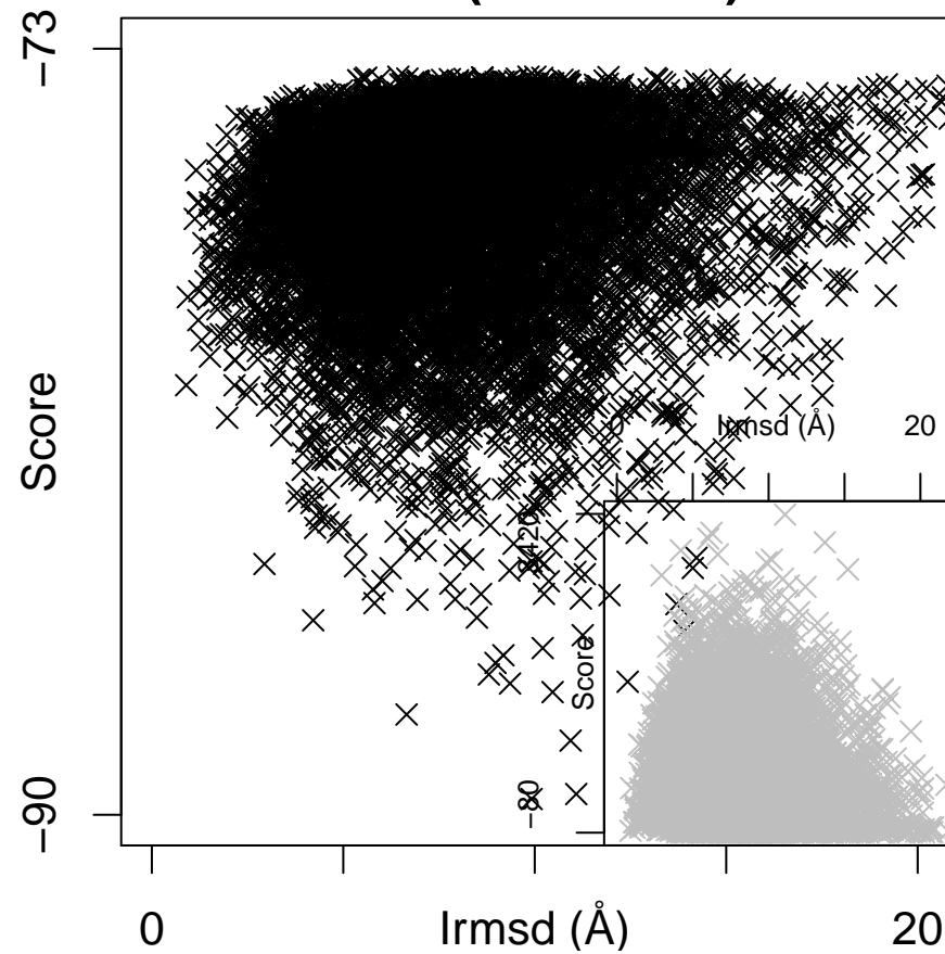
1g1x (ES = 0.54)
