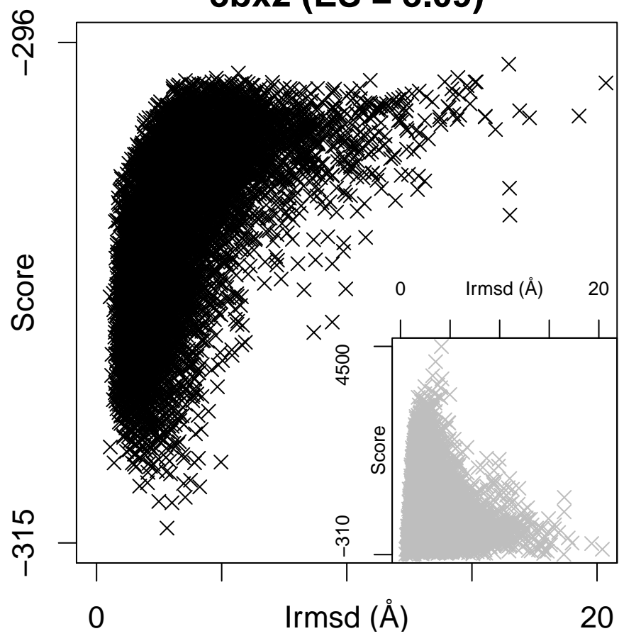
3bx2 (ES = 3.09)
