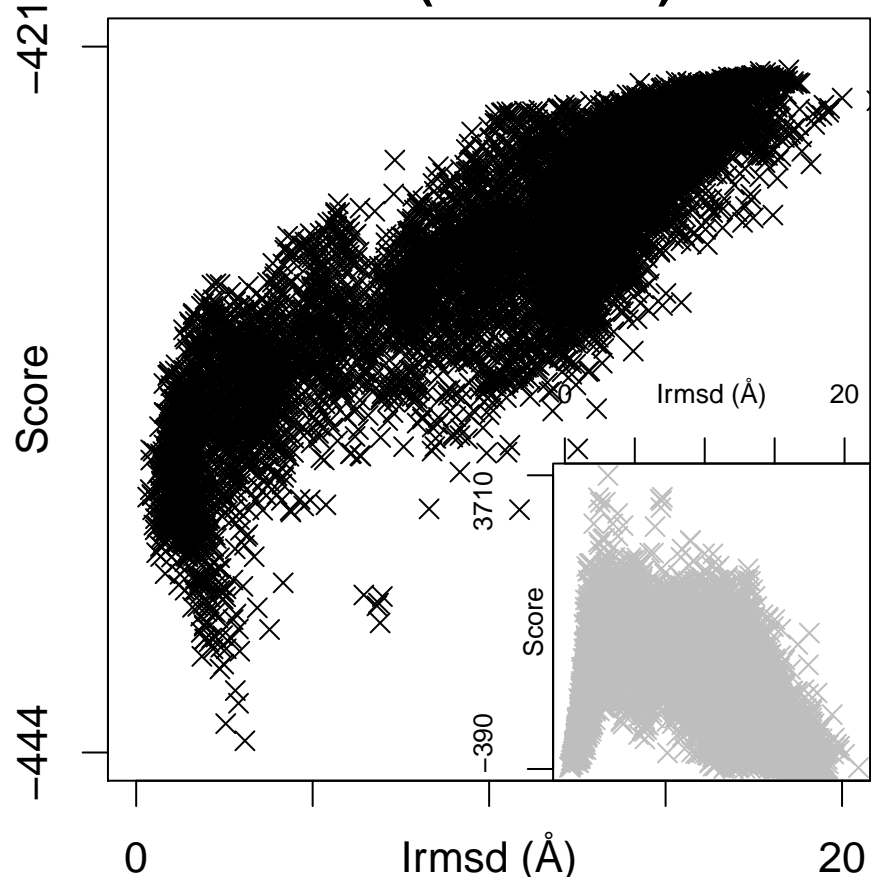
2i91 (ES = 7.35)
