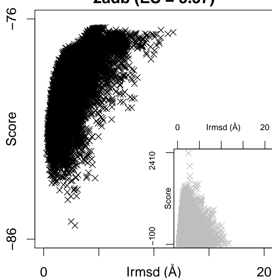
2adb (ES = 3.37)
