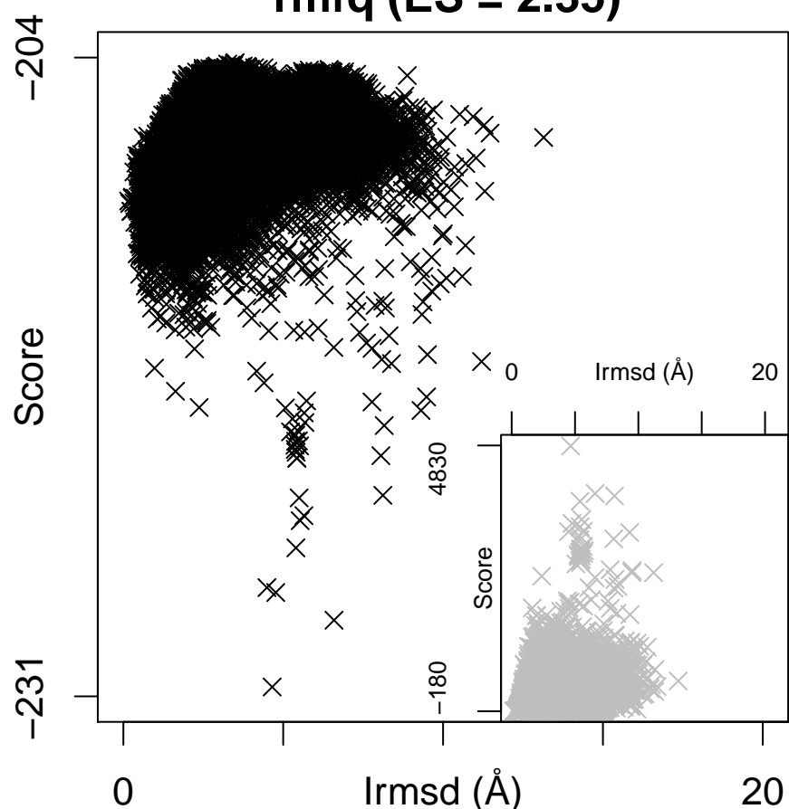
1mfq (ES = 2.35)
