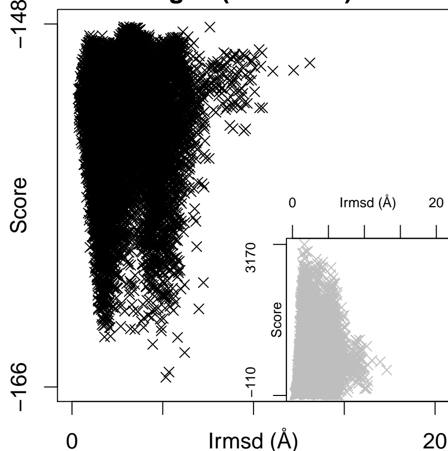
1g1x (ES = 0.54)
