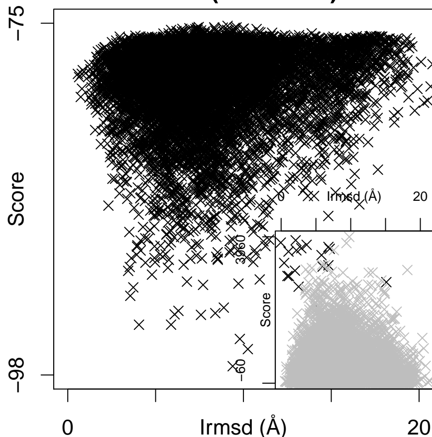
1ekz (ES = 0.81)
