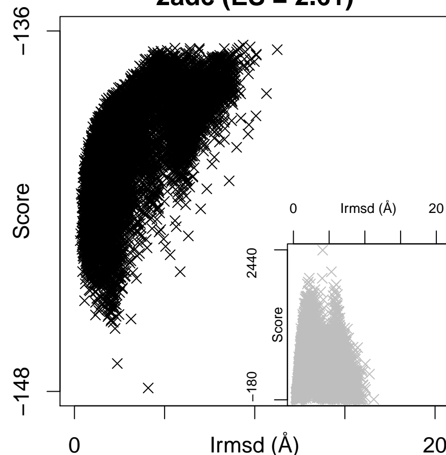
2adc (ES = 2.61)
