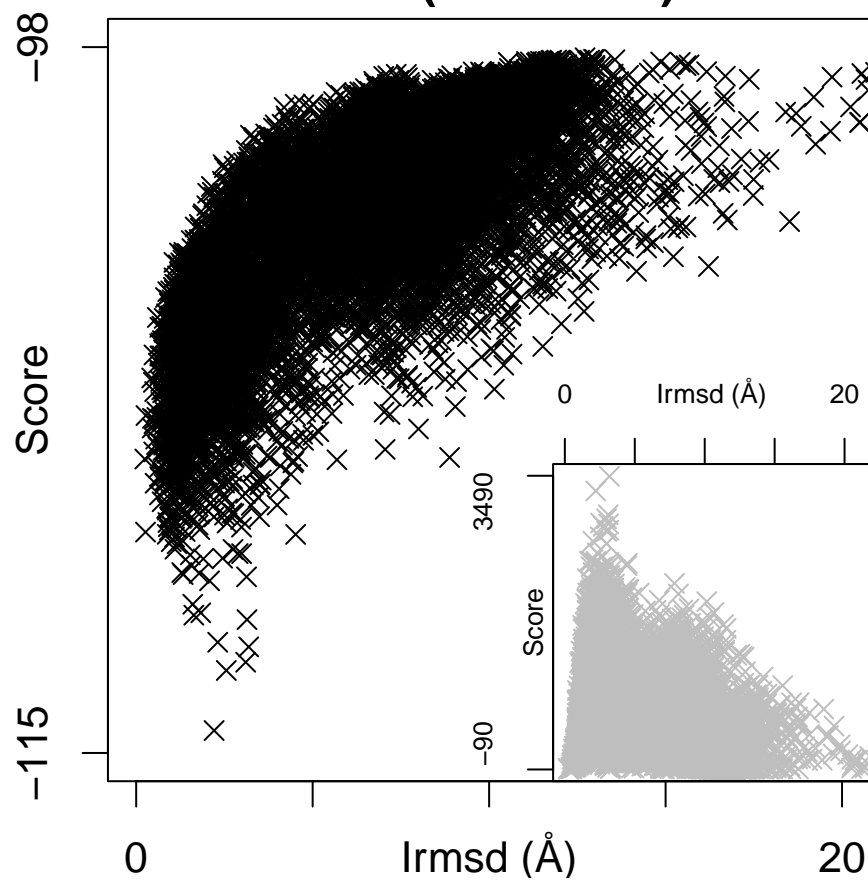
1e7k (ES = 1.33)
