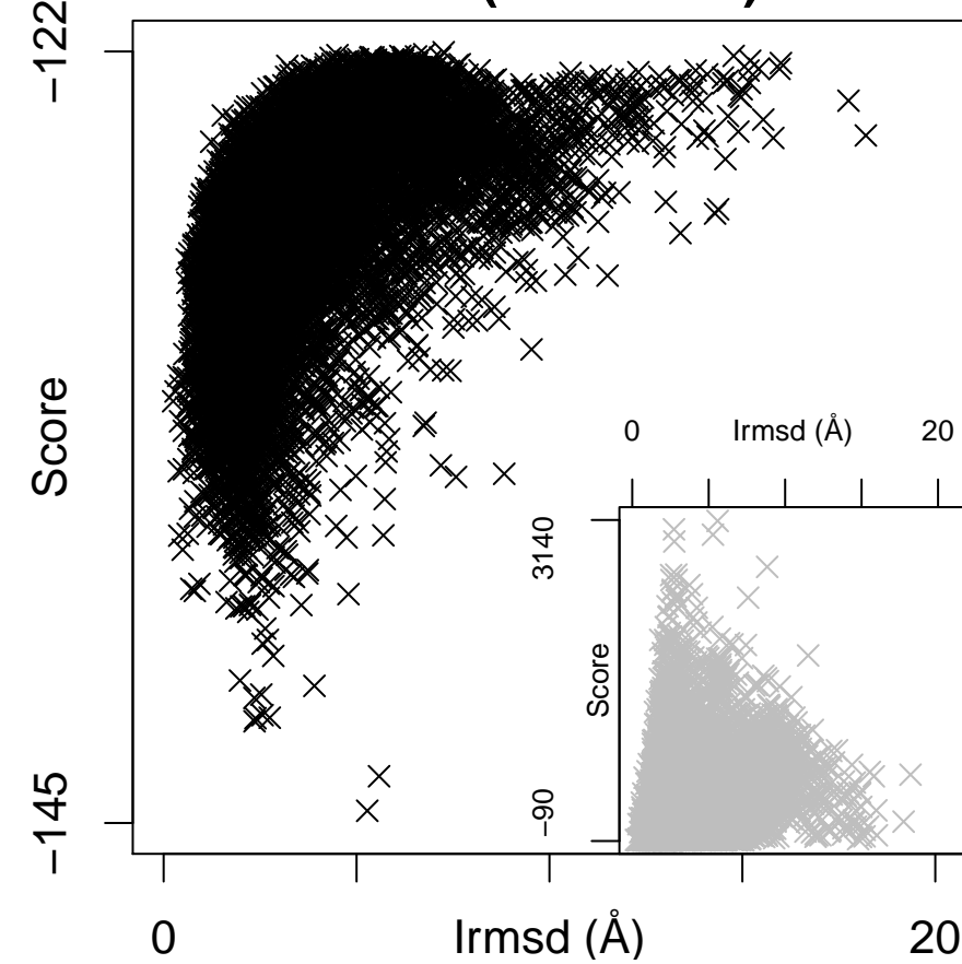
1efw (ES = 2.9)
