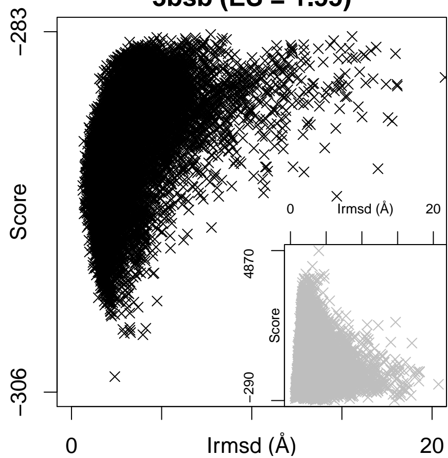
3bsb (ES = 1.55)
