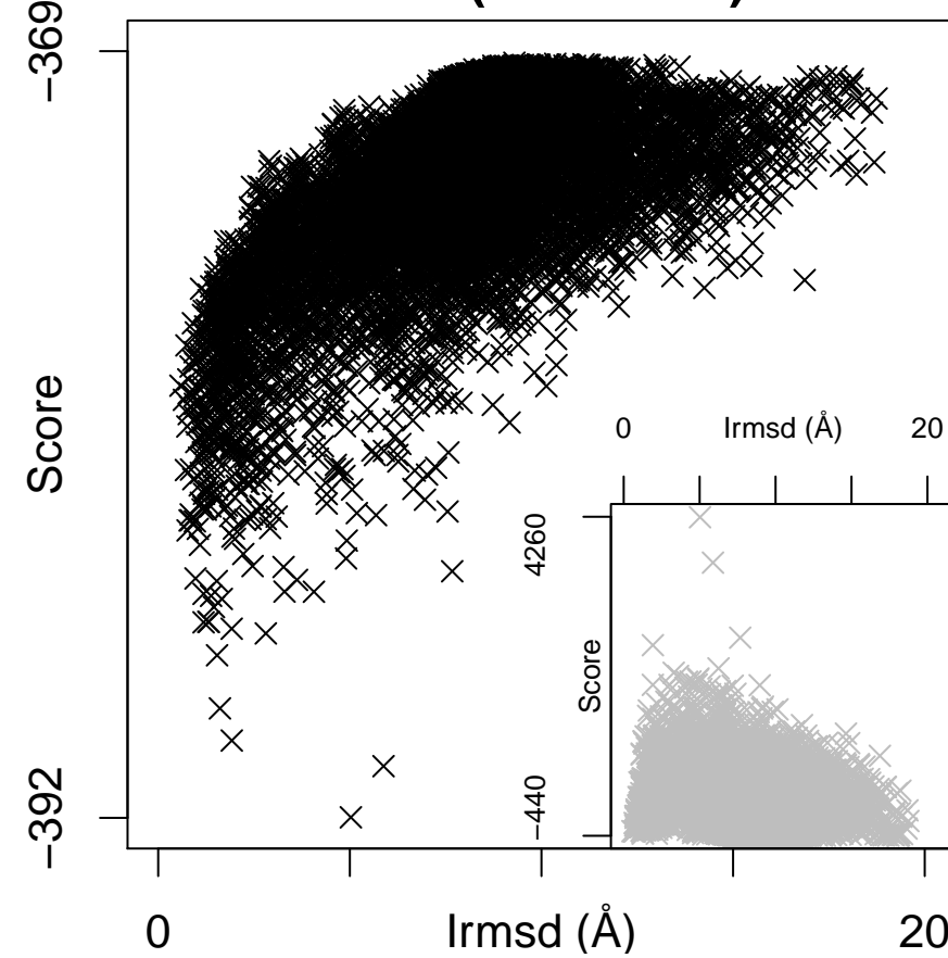
2hgh (ES = 1.03)
