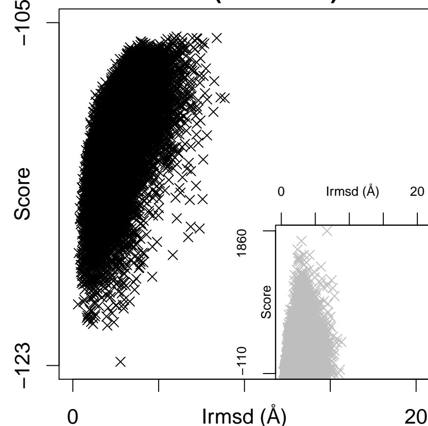
1hc8 (ES = 3.63)
