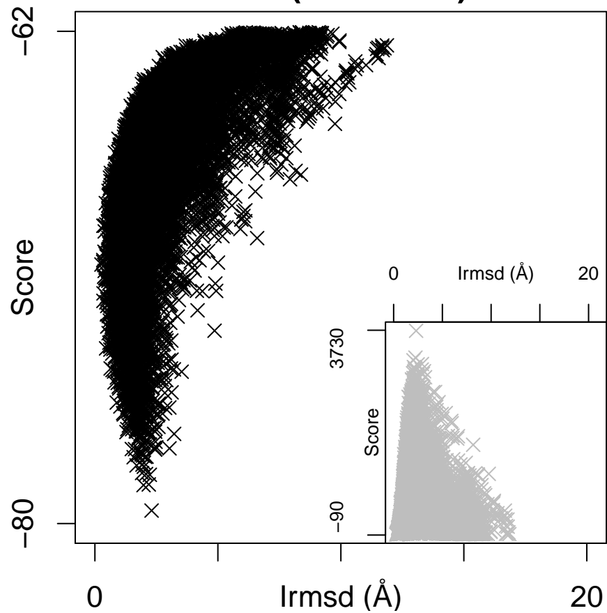
2i91 (ES = 7.35)
