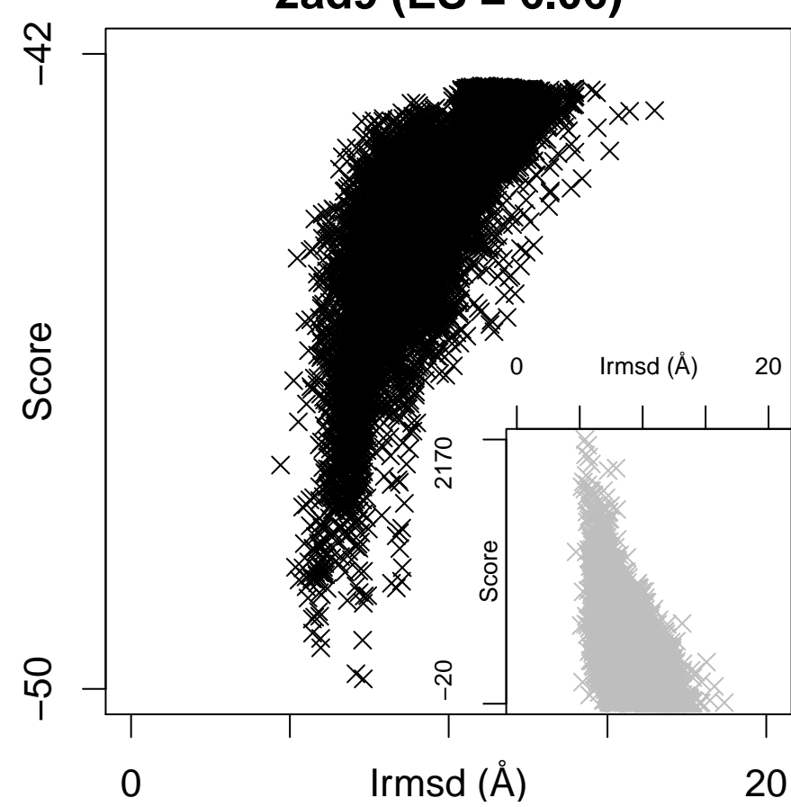
2ad9 (ES = 6.06)
