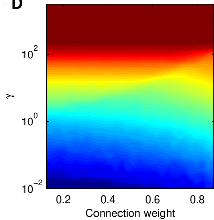
reg. lat.
