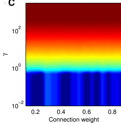
Erdős-Rényi
