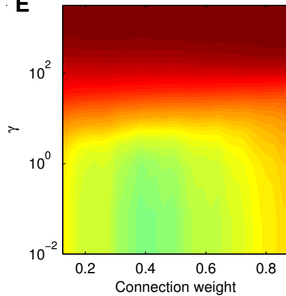
Brain DSI
