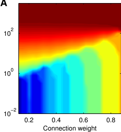
frac. hier.
