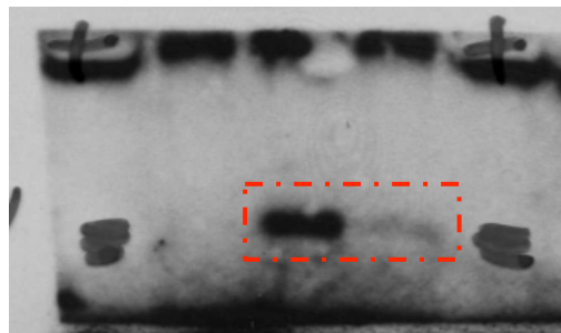
XIAP
