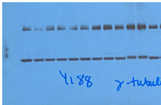
\gamma -tubulin
