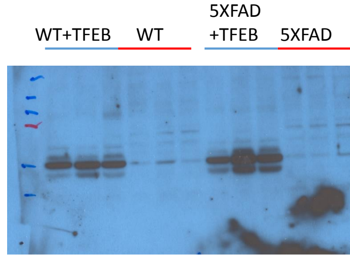
TFEB
