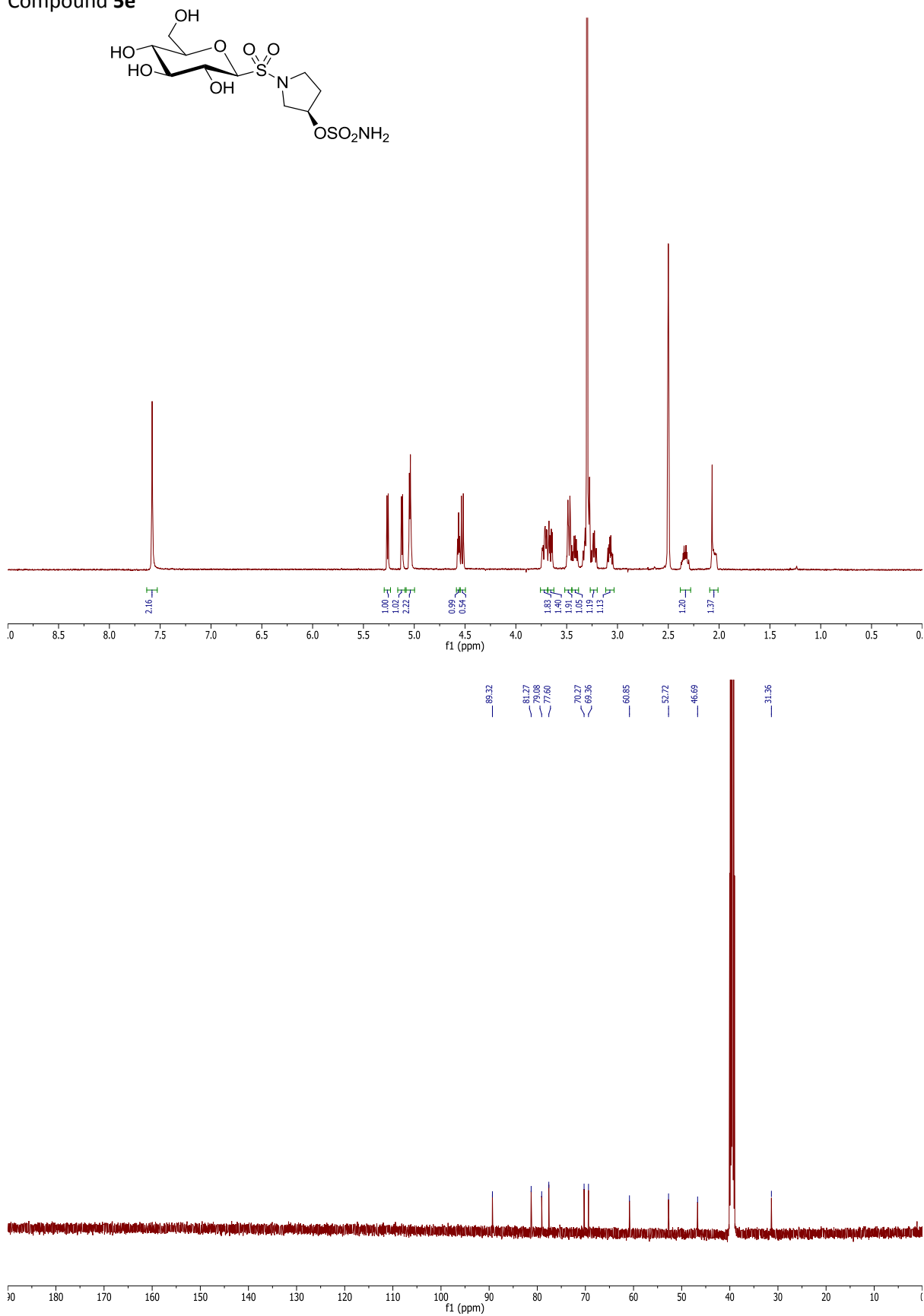
Compound 5e
