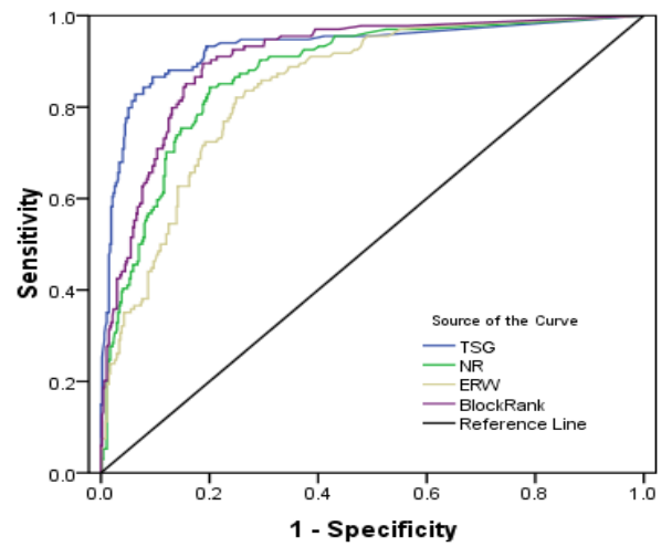
(d) ROC Curve - Diabetes Mellitus
