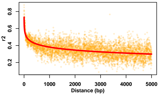
Chr1
