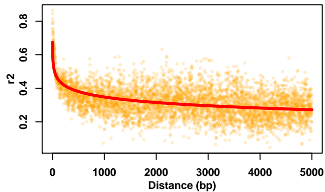
Chr4
