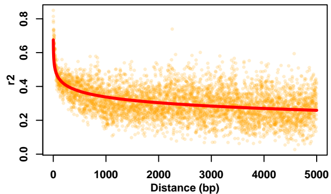
Chr10
