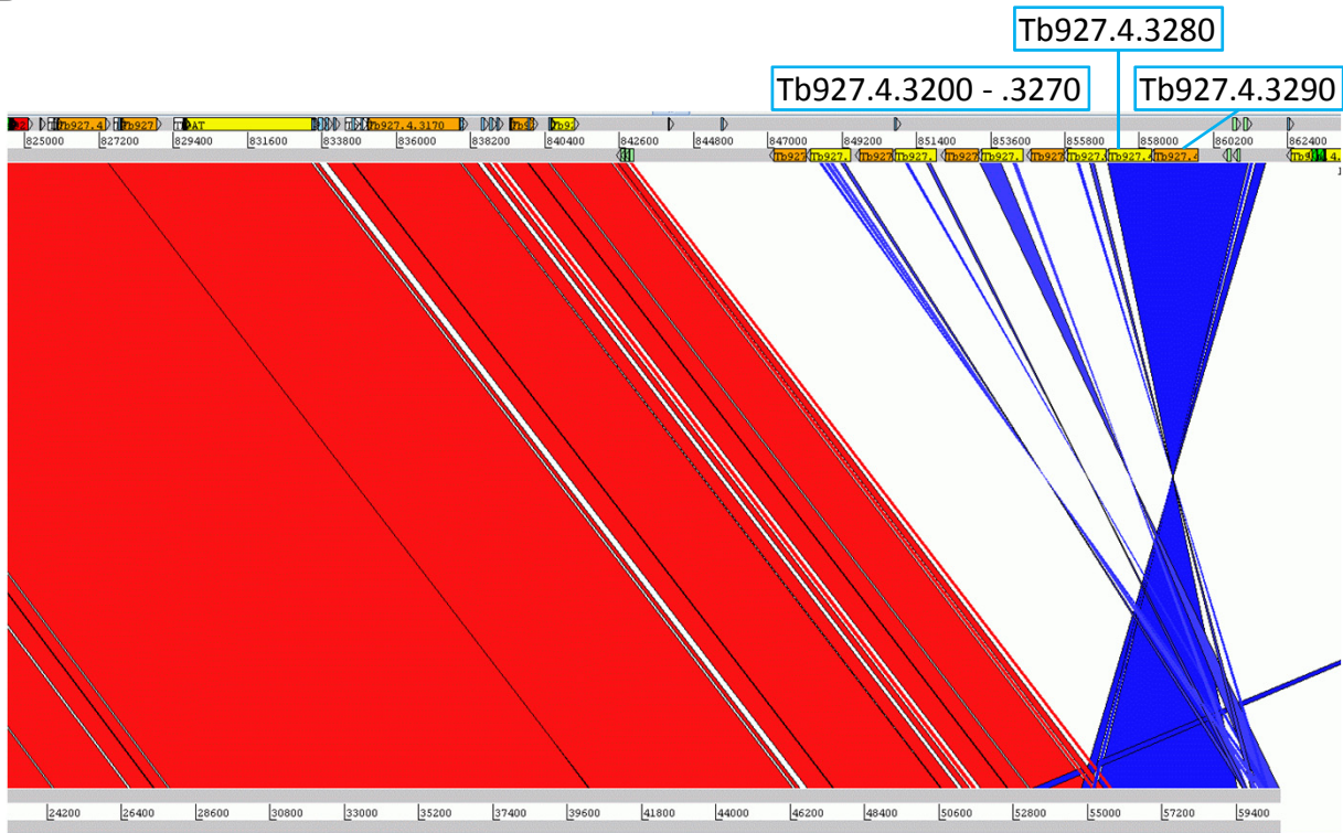
T. evansi STIB805 de novo contig
