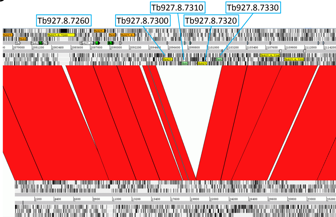
T. evansi STIB805 de novo contig
