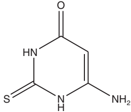
6 aminothiouracil
