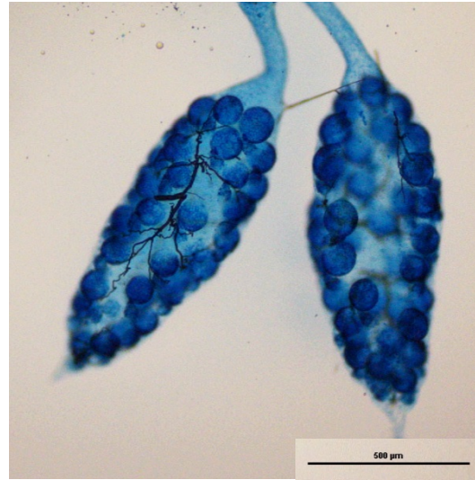
DMSO
