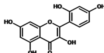
Morin
