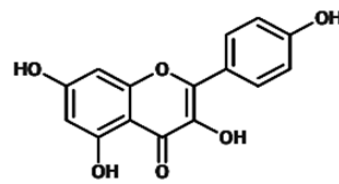
Kaempferol
