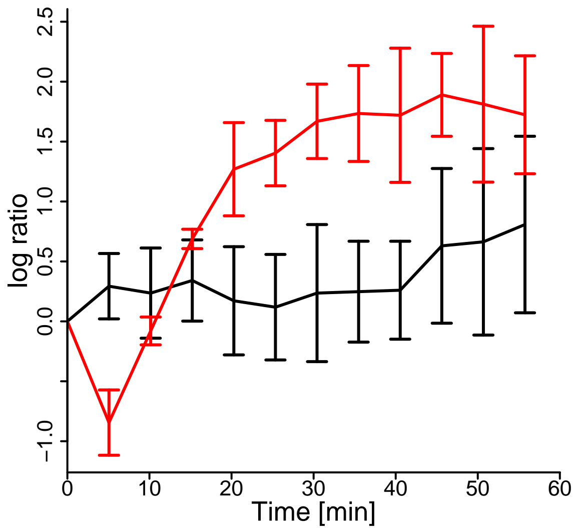
zntA( \Delta zur)
