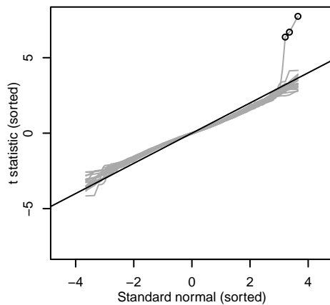
E. t(\text{Time0}) in S. oneidensis
