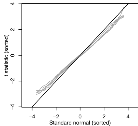
D. t(\text{Time0}) in S. amazonensis
