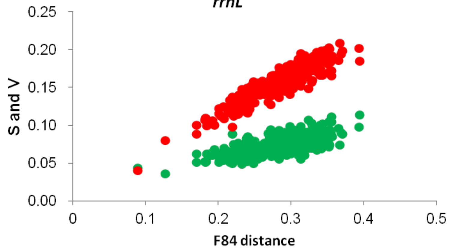
rrnL
