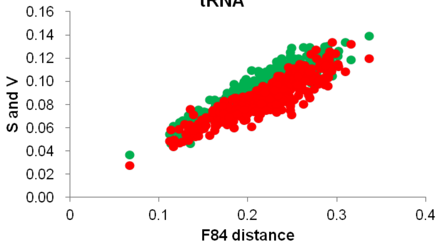
tRNA
