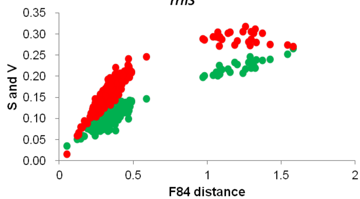
rrnS
