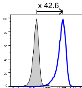
CD19+ K562
