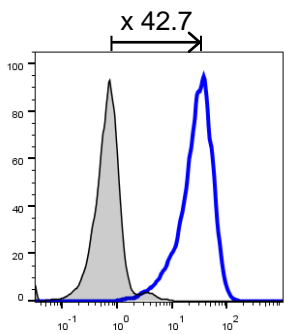
CD19+ H9
