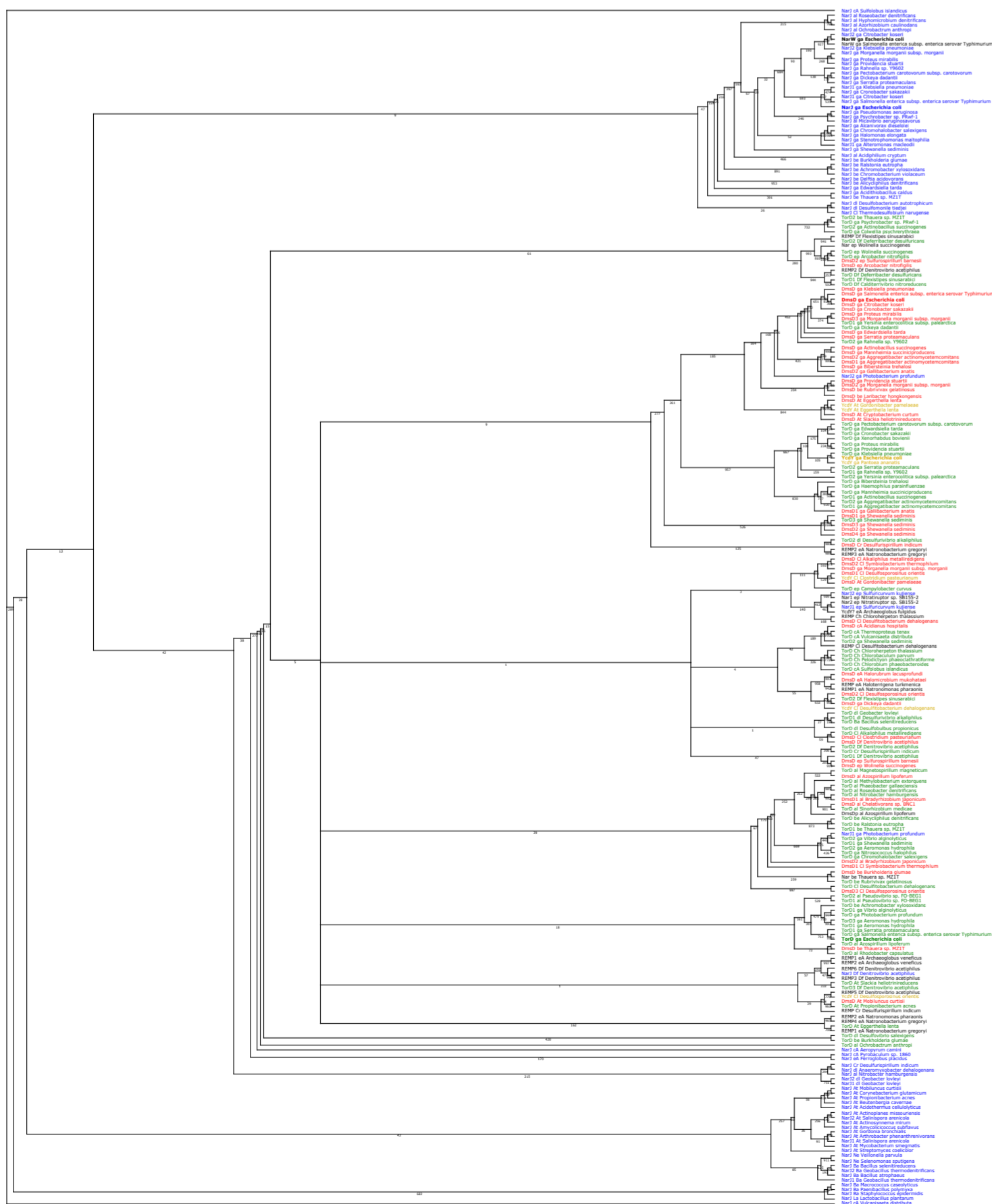
NarJ-NJ
