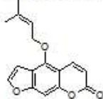
Isoimperatorine
