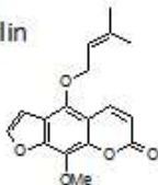
Isoimperatorine
