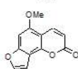
Isobergapten
