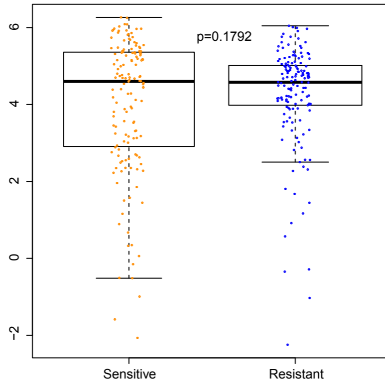
PF-2341066
