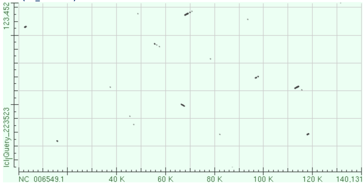
SGIV (NC_006549.1)-SDDV
