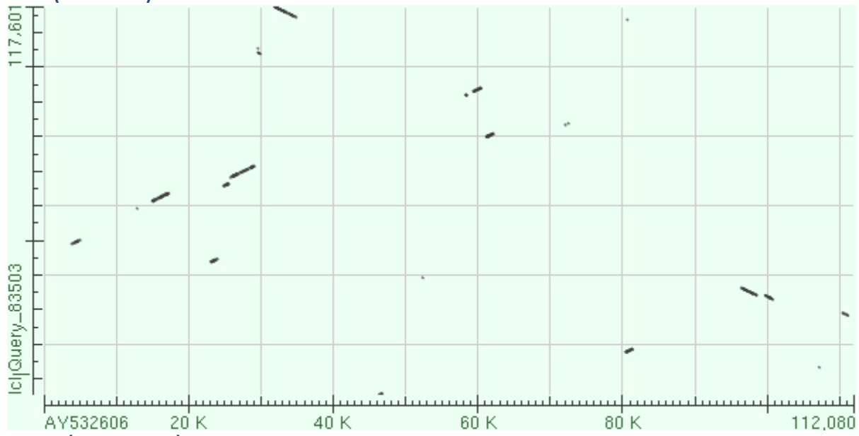
OSGIV (AY894343.1)-SDDV
