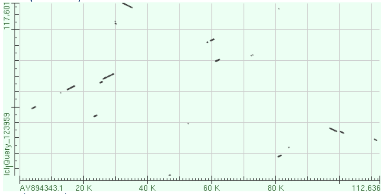
RSIV (BD143114)-SDDV
