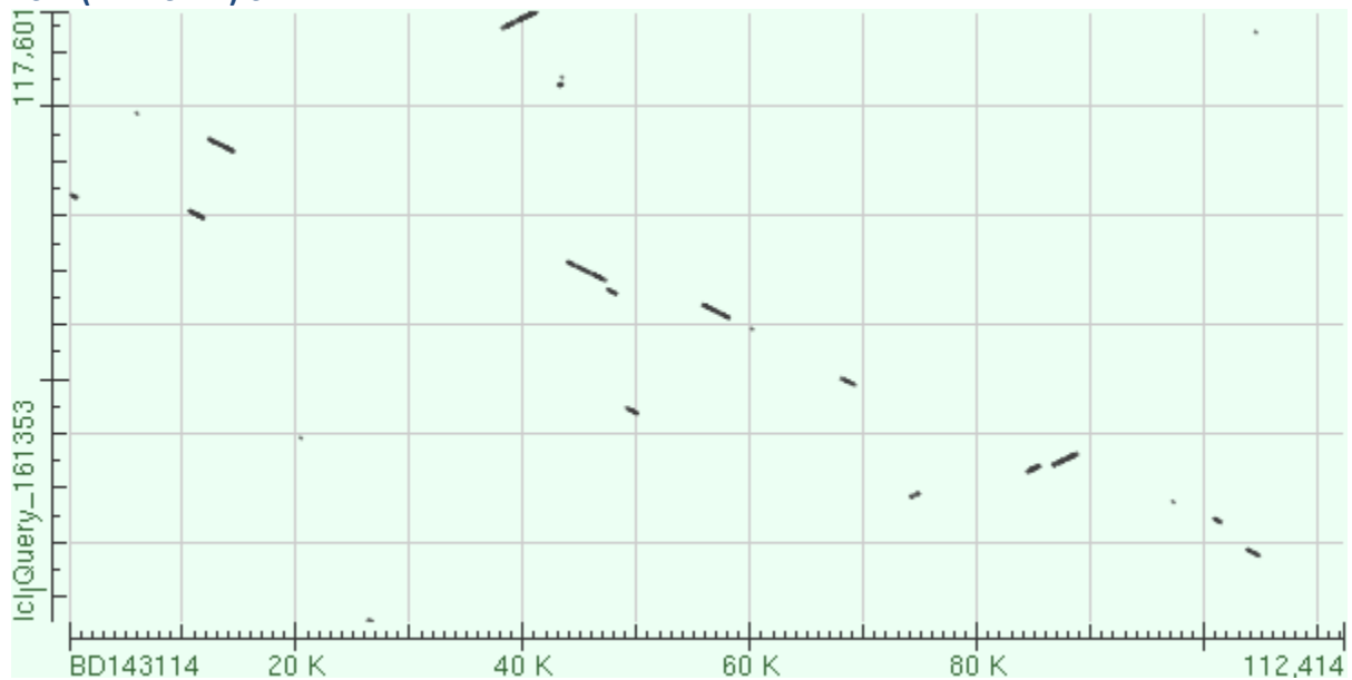
RSIV (BD143114)-SDDV
