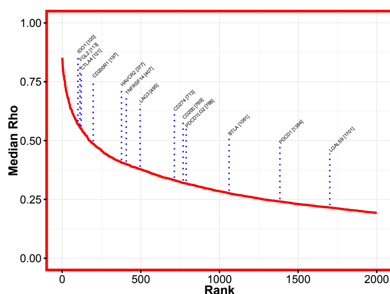
TRAT1
