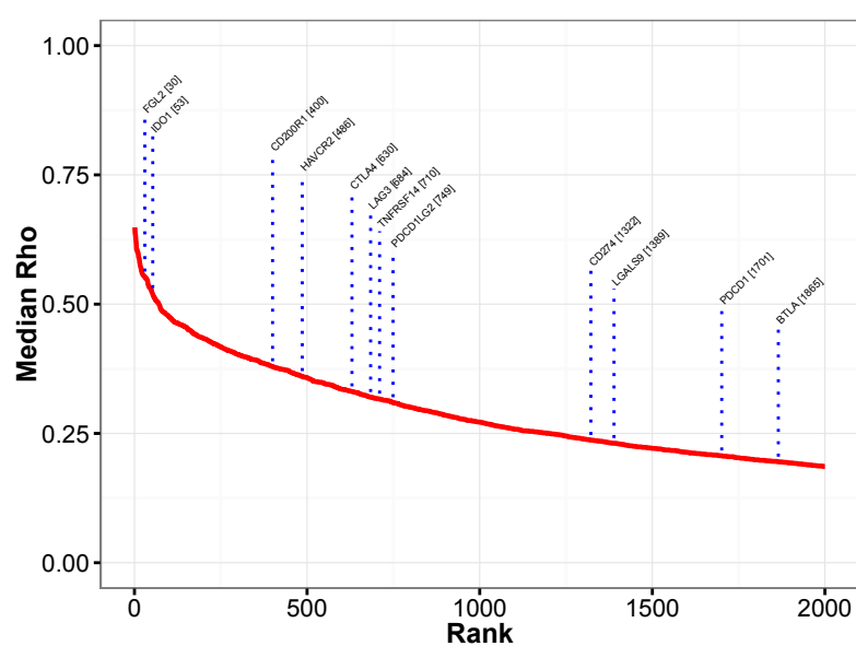
GZMK
