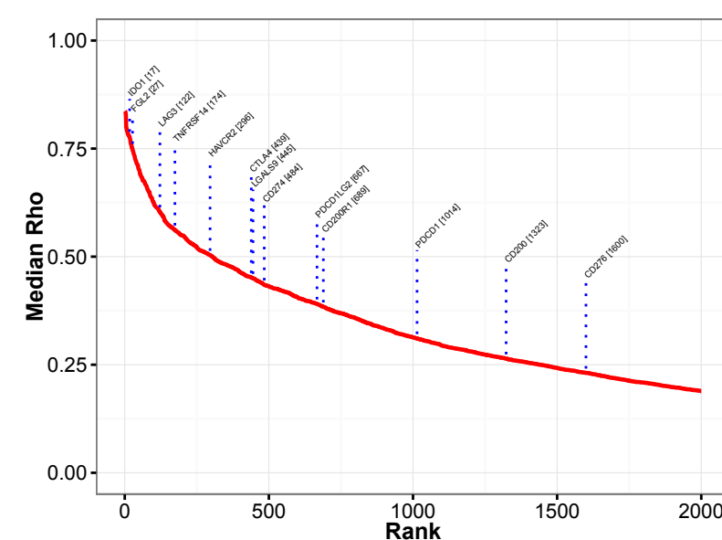
UBASH3A
