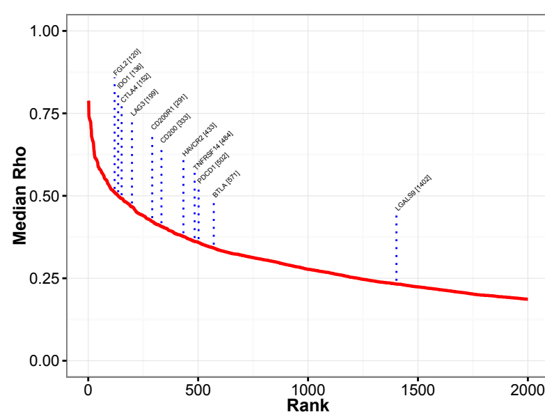
TRBC1
