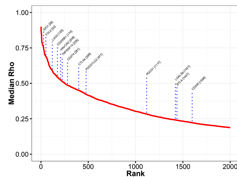
RARRES3
