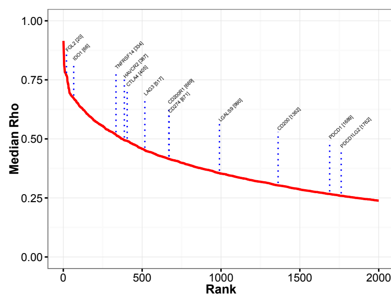
ITM2A
