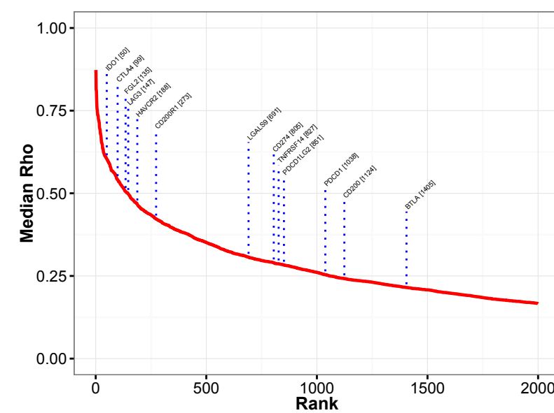
GZMA
