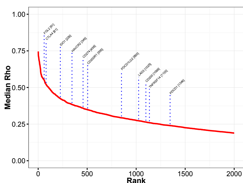
TCN2
