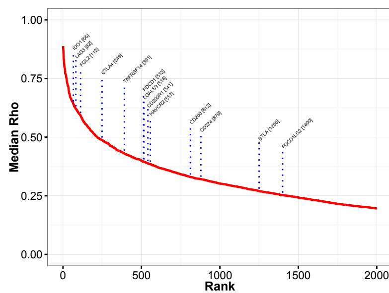
GIMAP6
