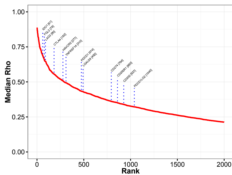
FGL2
