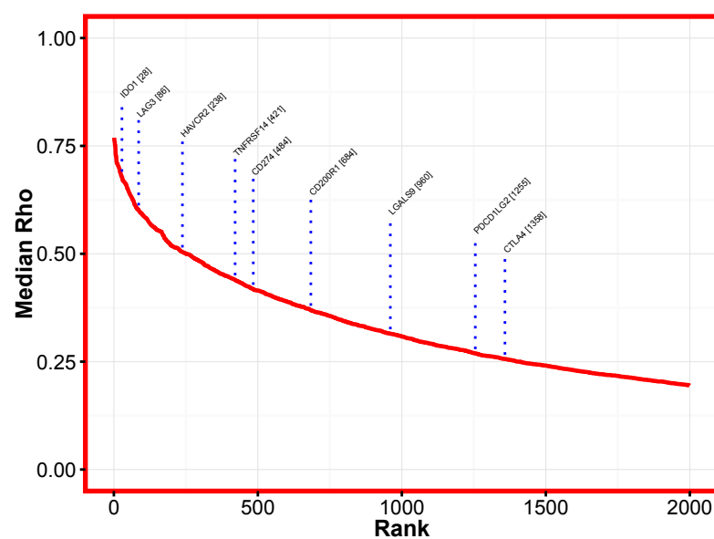
IFNG
