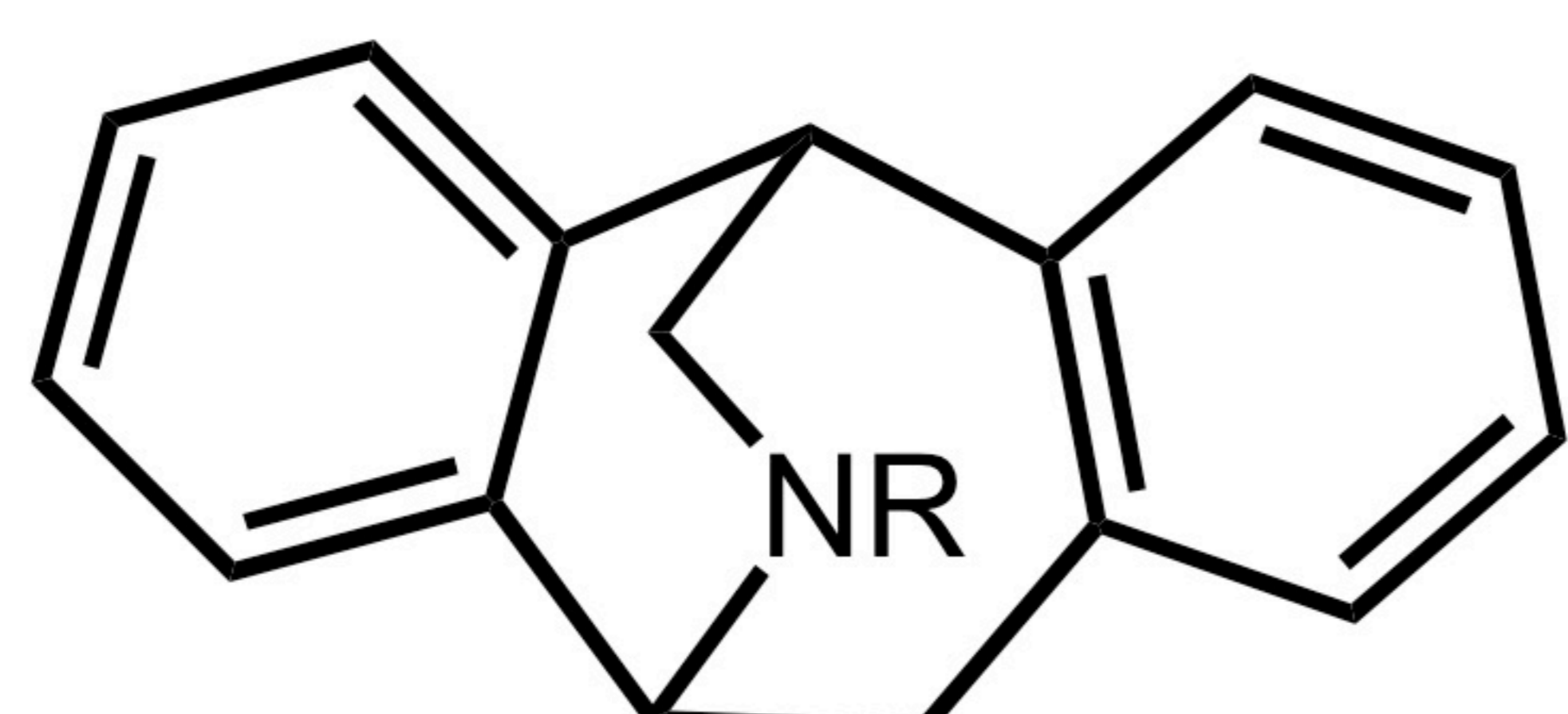
Isopavine
