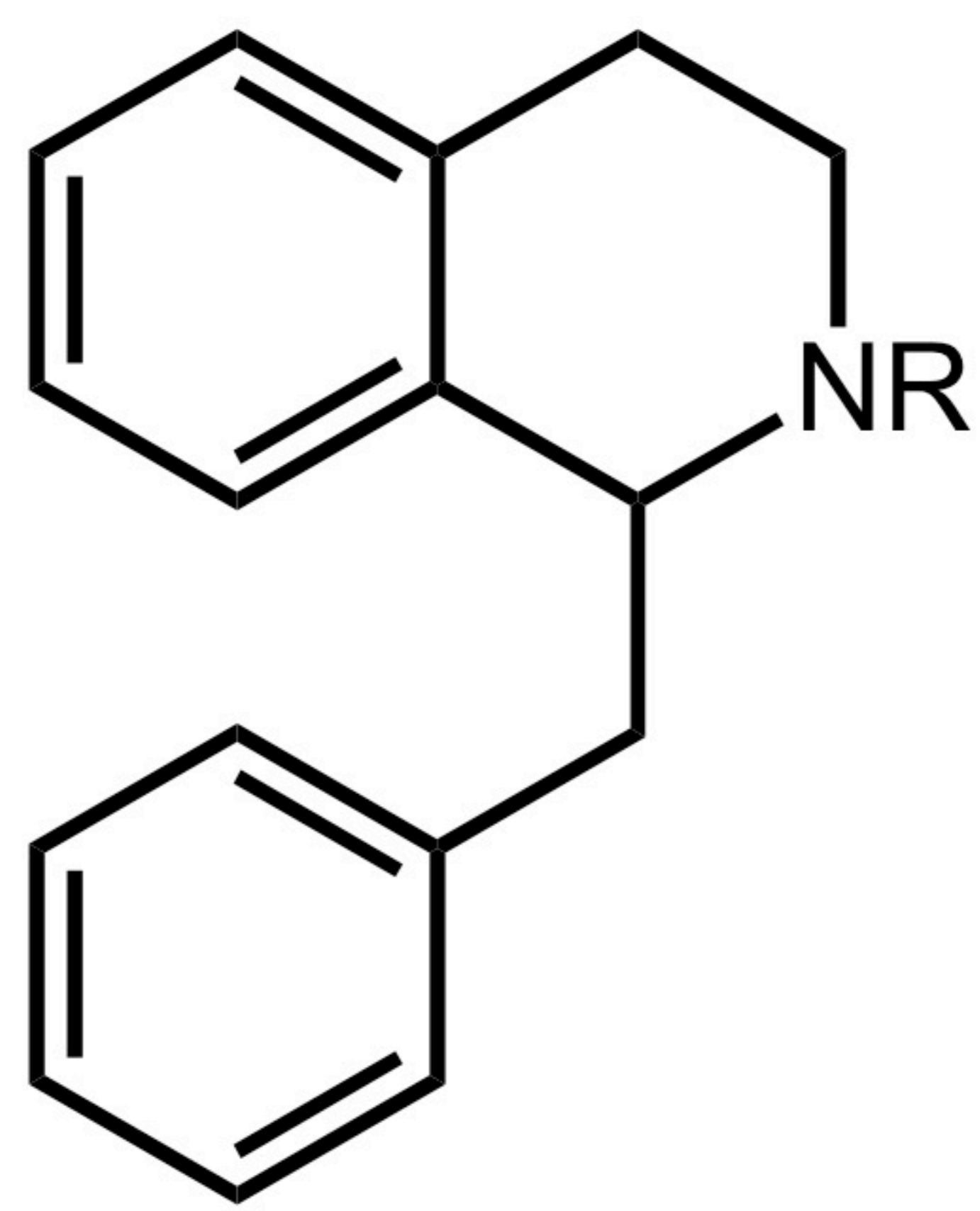
1-Benzylisoquinoline
