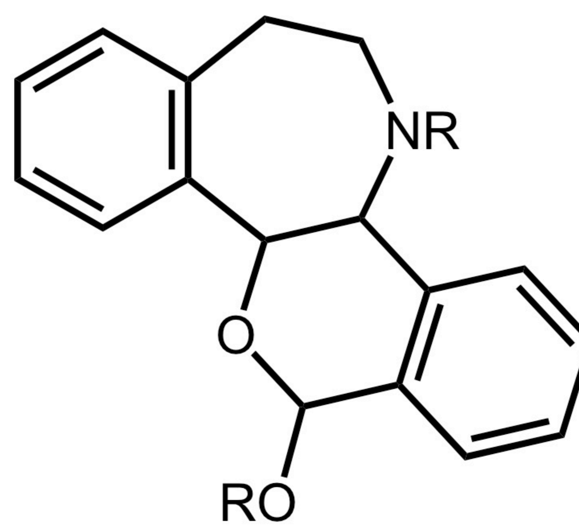
Papaverubine
