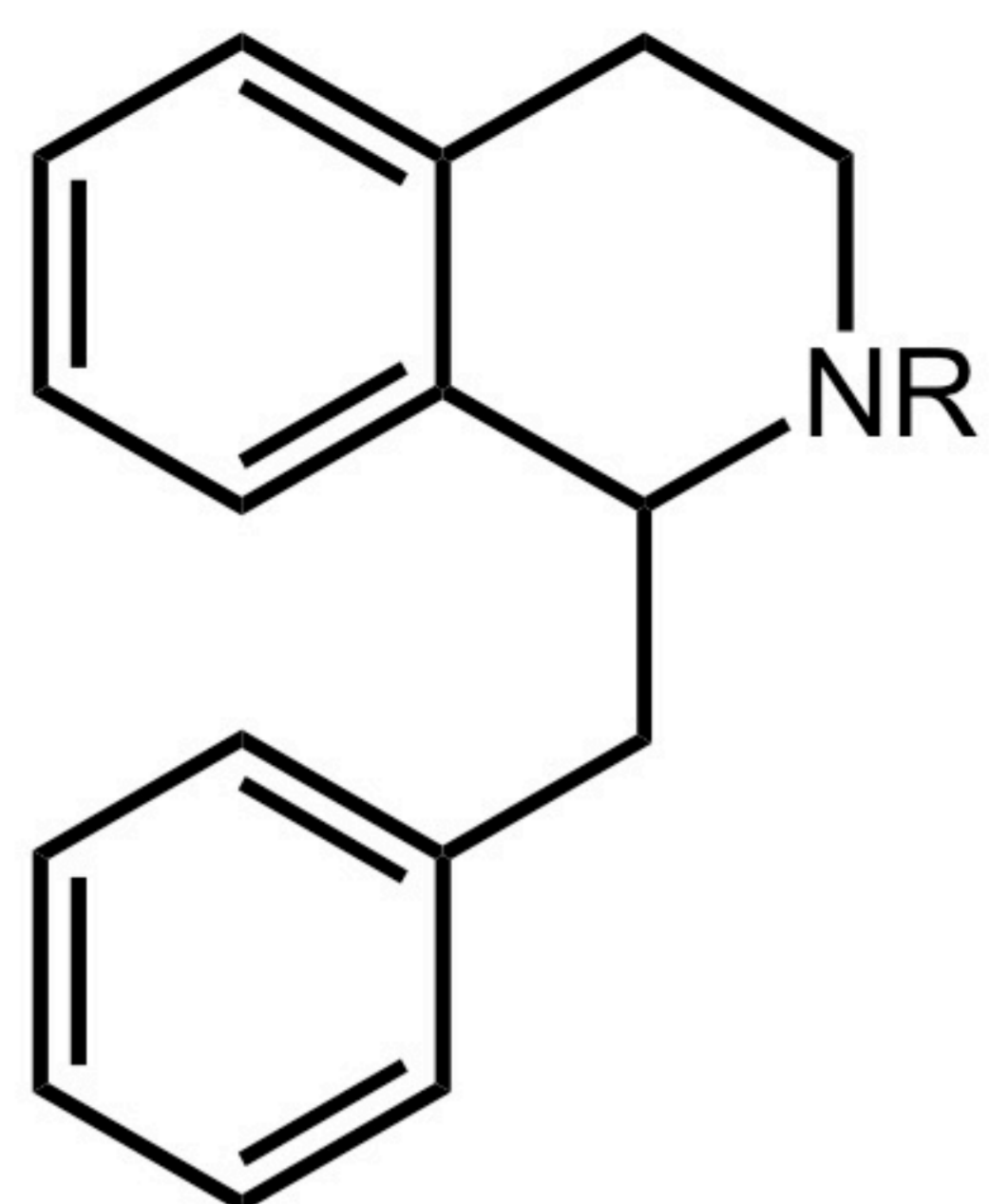
1-Benzylisoquinoline
