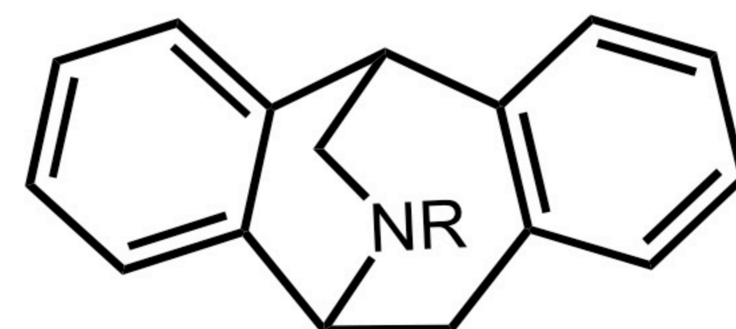
Isopavine
