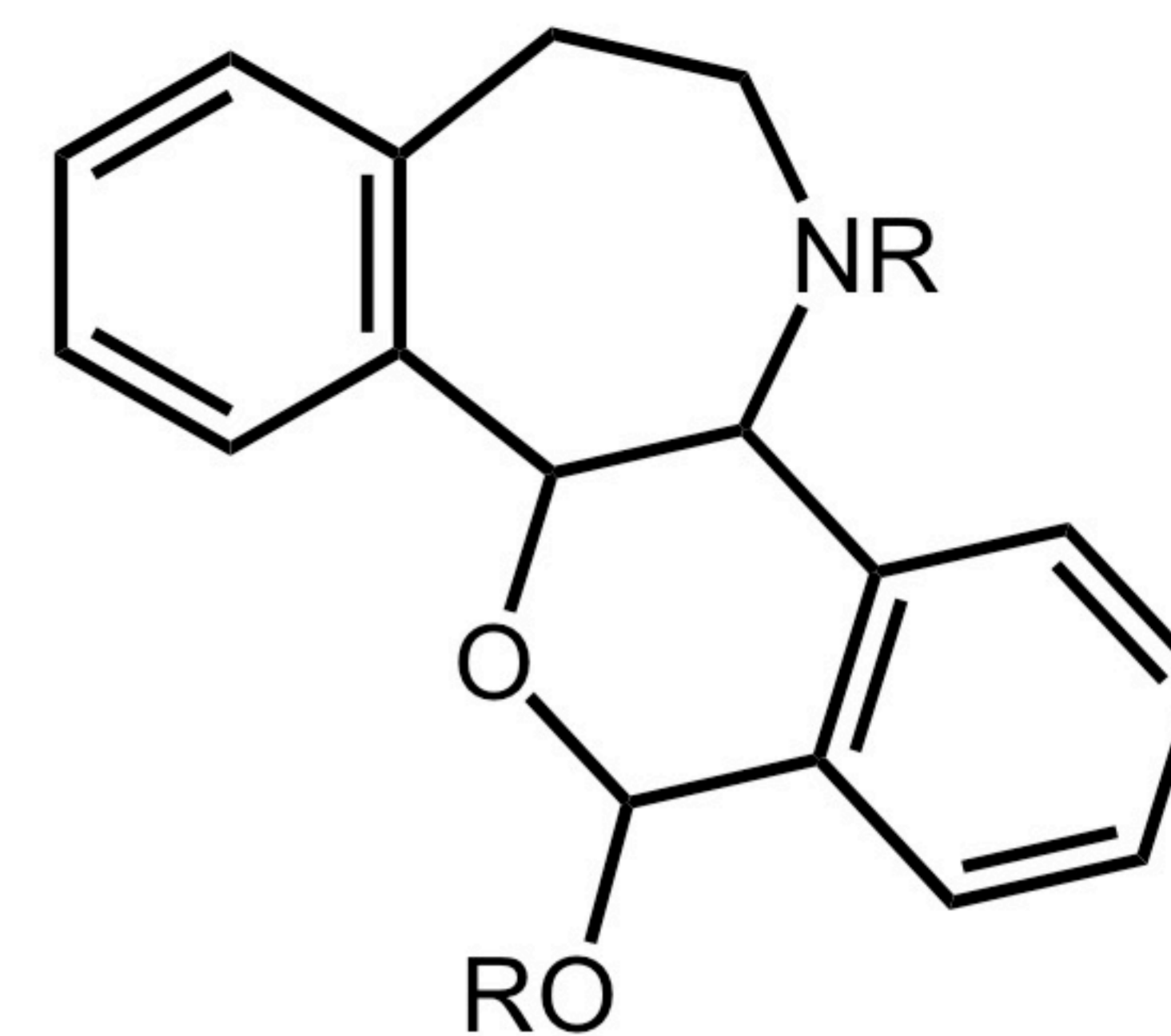
Papaverubine
