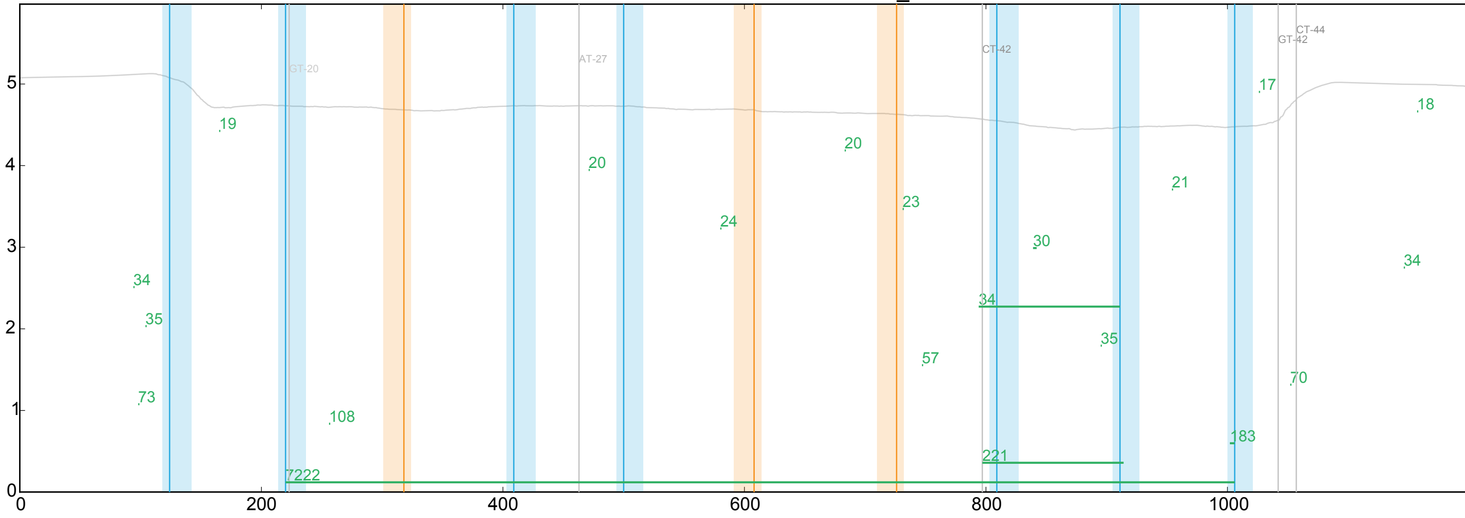
WT ENSDARG00000078582_31
