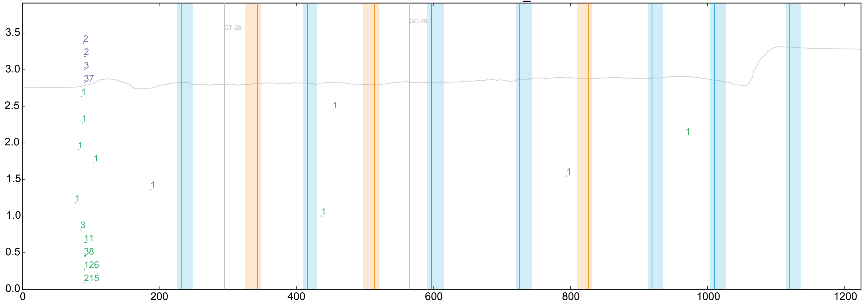
WT ENSDARG00000057792_1
