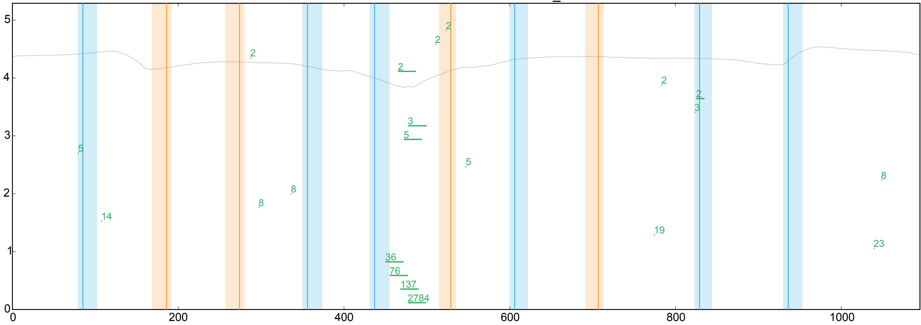
WT ENSDARG00000079969_4
