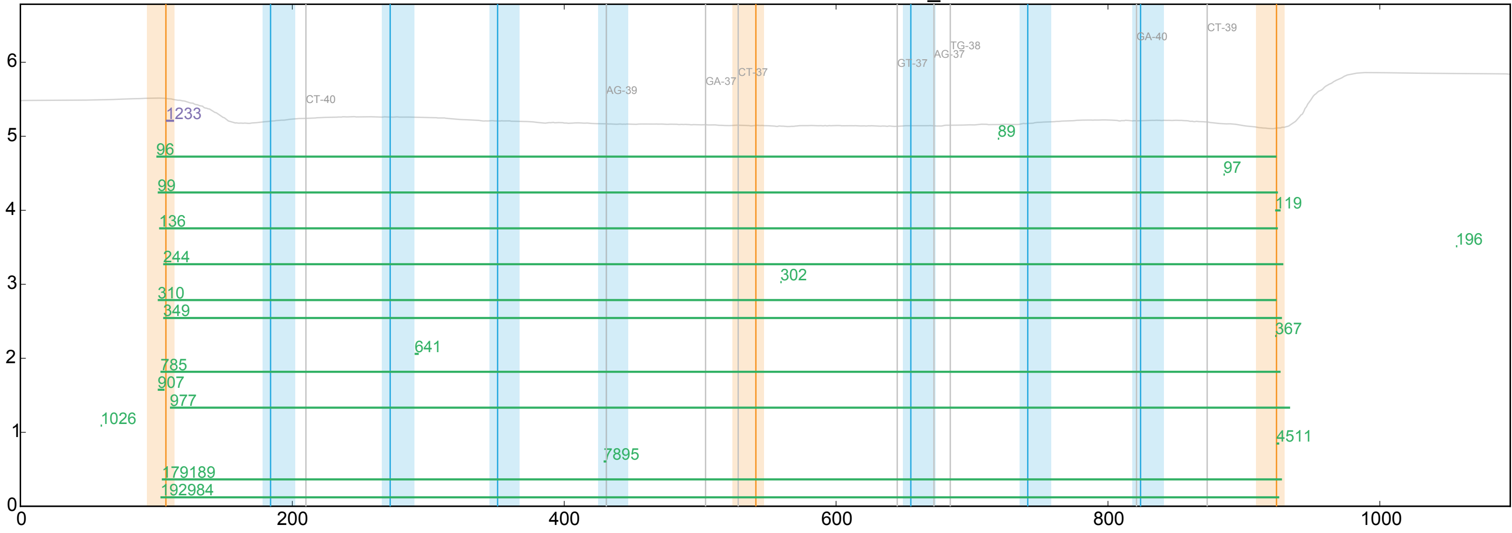
WT ENSDARG00000068650_6
