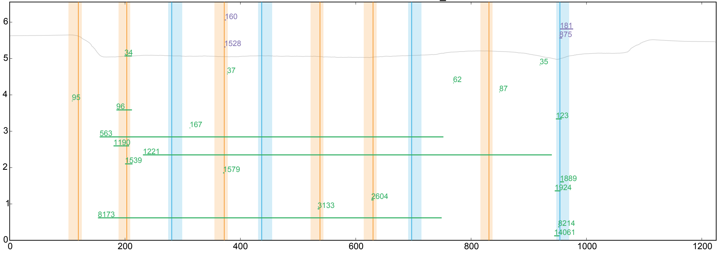
WT ENSDARG00000074919_0
