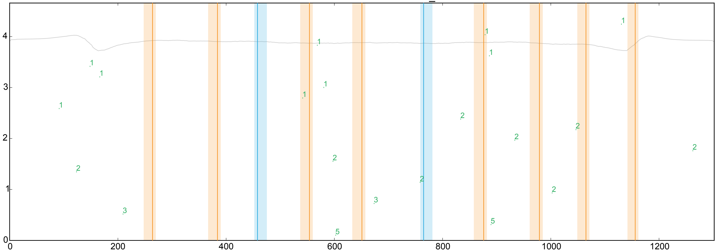
WT ENSDARG0000004377_4
