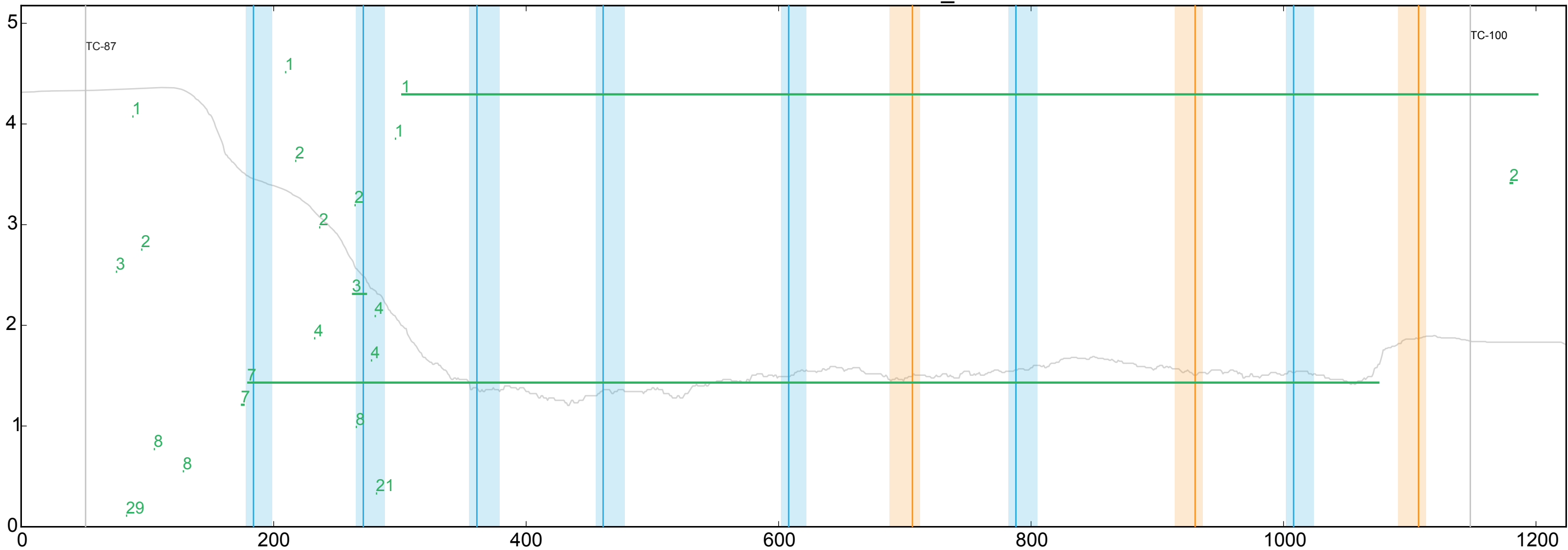
WT ENSDARG00000092067_5
