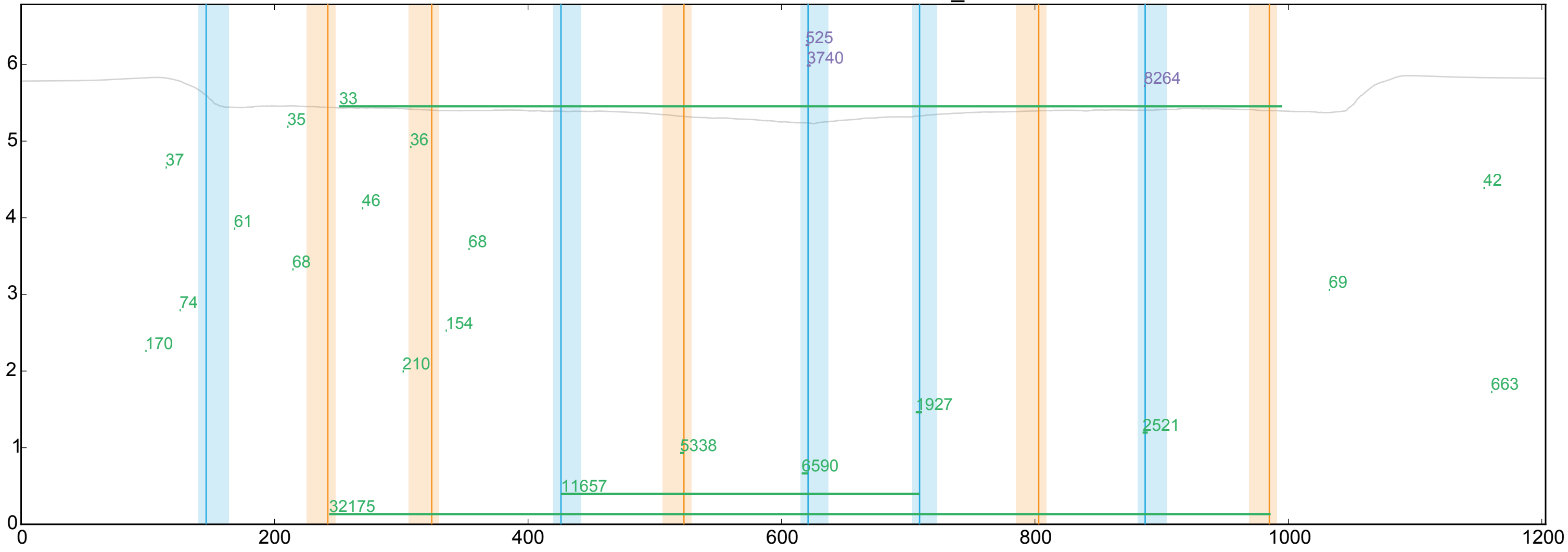
WT ENSDARG00000043246_3
