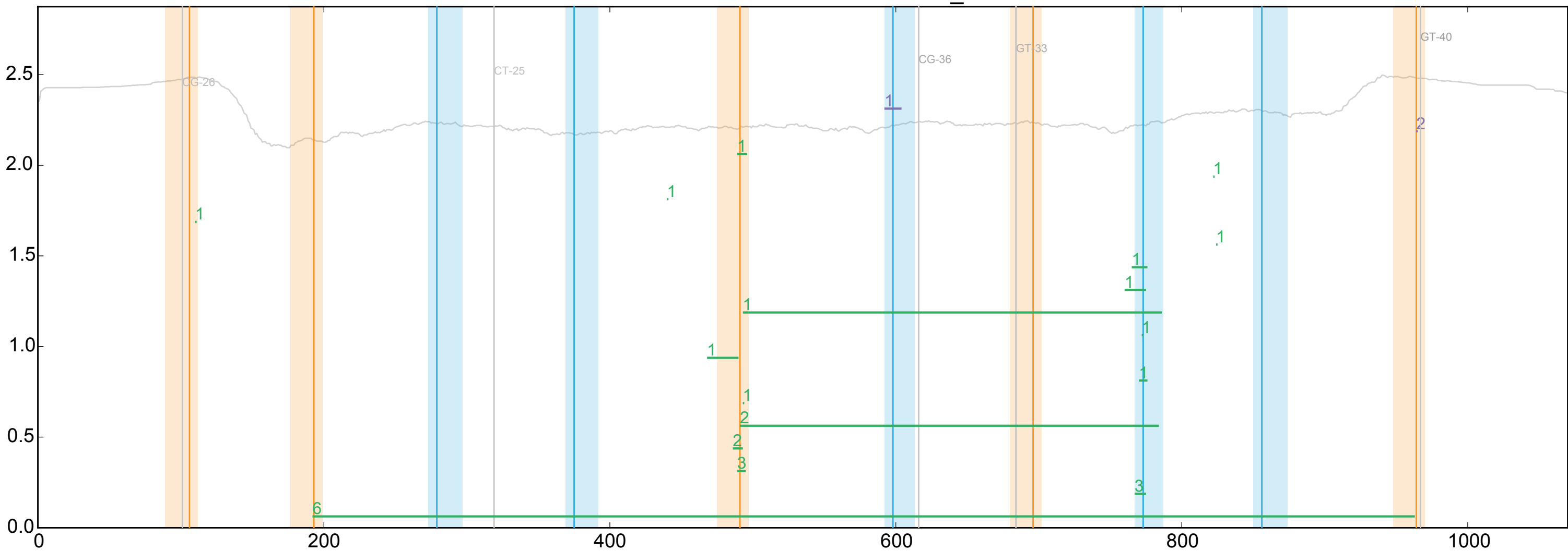
WT ENSDARG00000052232_0
