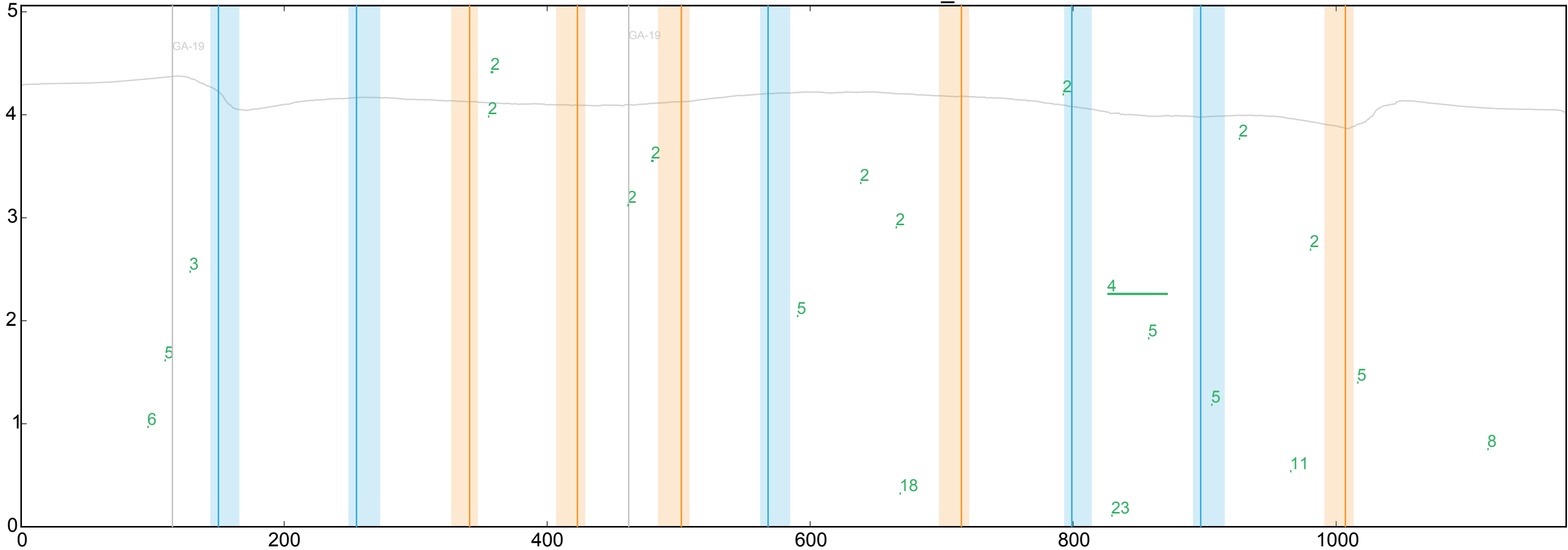
WT ENSDARG0000025108_6
