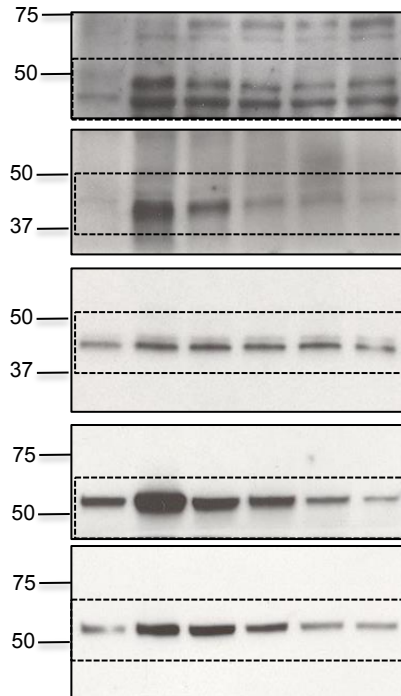
Fig. S4c (IMR90)
