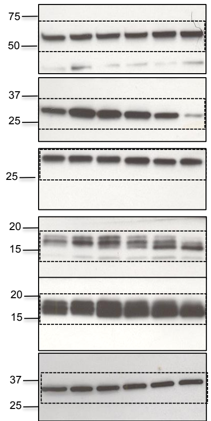
Fig. S4c (IMR90)
