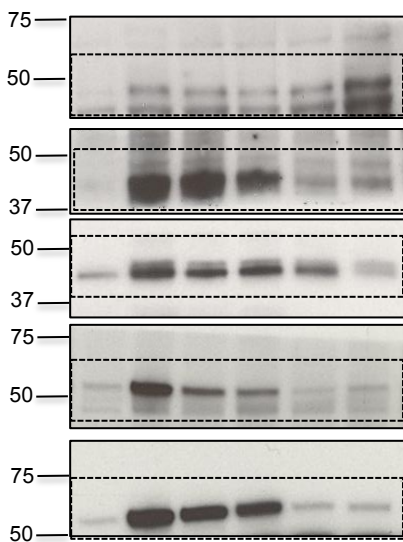
Fig. S4c (BJ)
