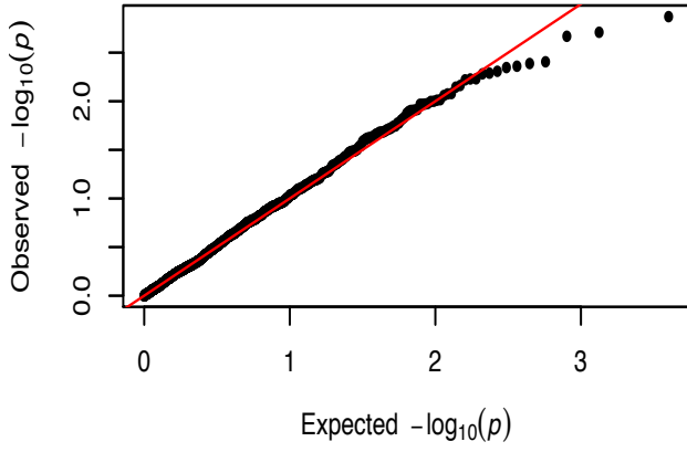
single trait
