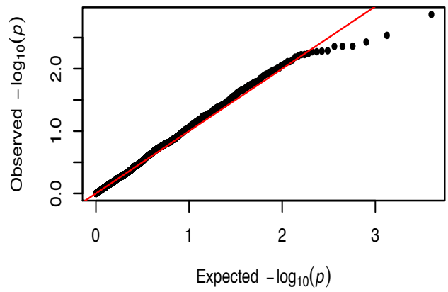
CCA
