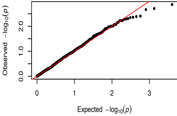
single trait
