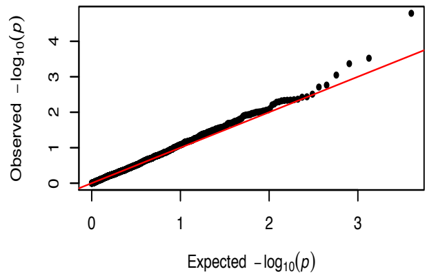
EN
