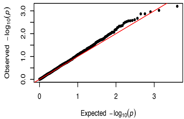
CCA
