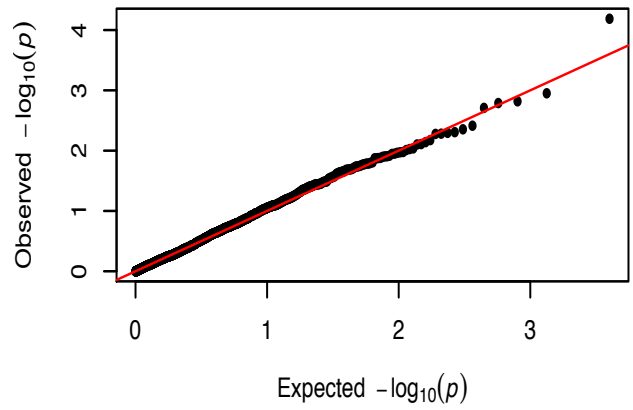
EN
