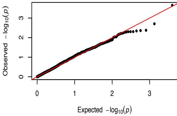
LM
