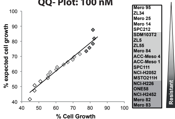
GDC-0980 QQ- Plot: 100 nM
