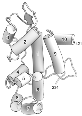
SaCas9
