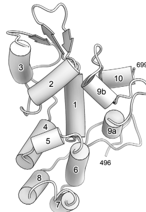
SpCas9
