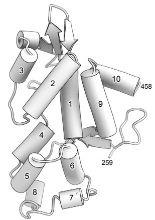
AnCas9
