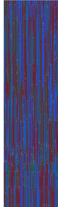
Chr11
