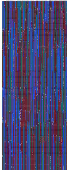
Chr10
