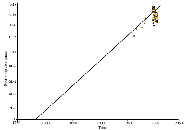
NS5 gene
