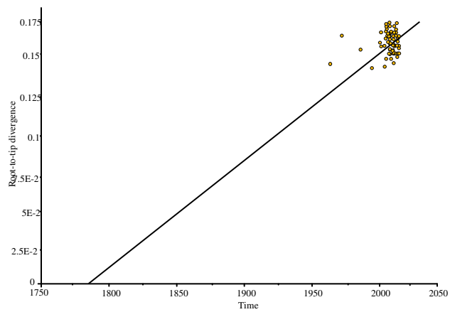
E gene
